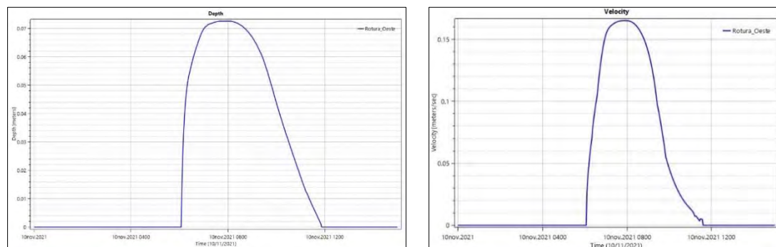
Ilustración 268.- Gráficos de calado y velocidad en el punto de la carretera LE-6605 afectado por la rotura de la balsa S-II.
