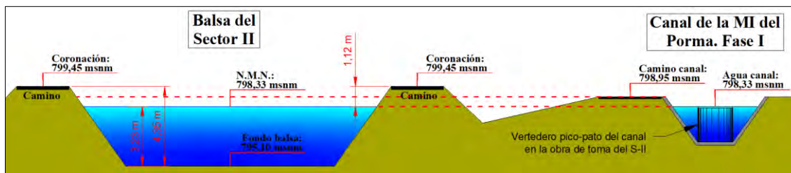
Ilustración 237.- Esquema de cotas de la balsa del S-II y del Canal de la MI del Porma, Fase I.
