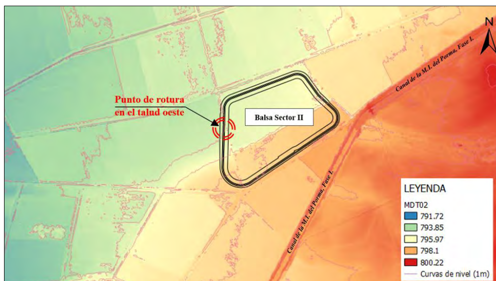
Ilustración 238.- Estudio de rotura de la balsa del S-II. Ubicación del punto de rotura.
