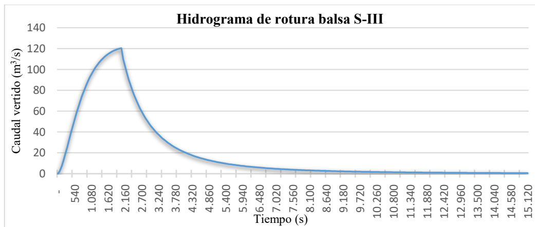
Ilustración 277.- Hidrograma de rotura para la simulación de la balsa del S-III.
