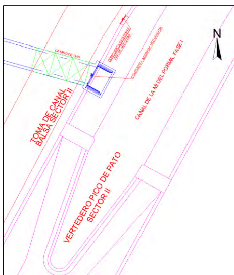
Ilustración 21.- Vista en planta de la obra de toma a balsa del sector II aguas arriba del pico-pato.
