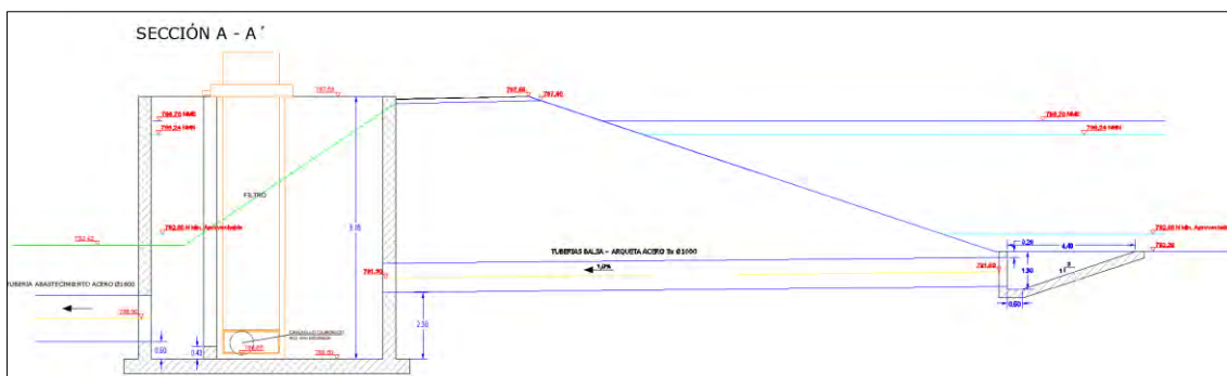
Ilustración 33.- Vista en sección de la toma en balsa, tuberías de acero y arqueta de filtros del sector III.
