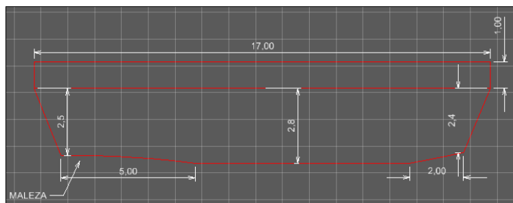
Ilustración 261.- Geometría del puente de la FFCC de alta velocidad Venta de Baños-León sobre el Arroyo Valdearcos.
