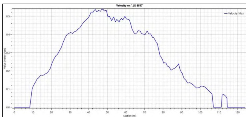
Ilustración 296.- Gráfico de velocidad máxima en la afección n.º 3 sobre la carretera LE-6617.
