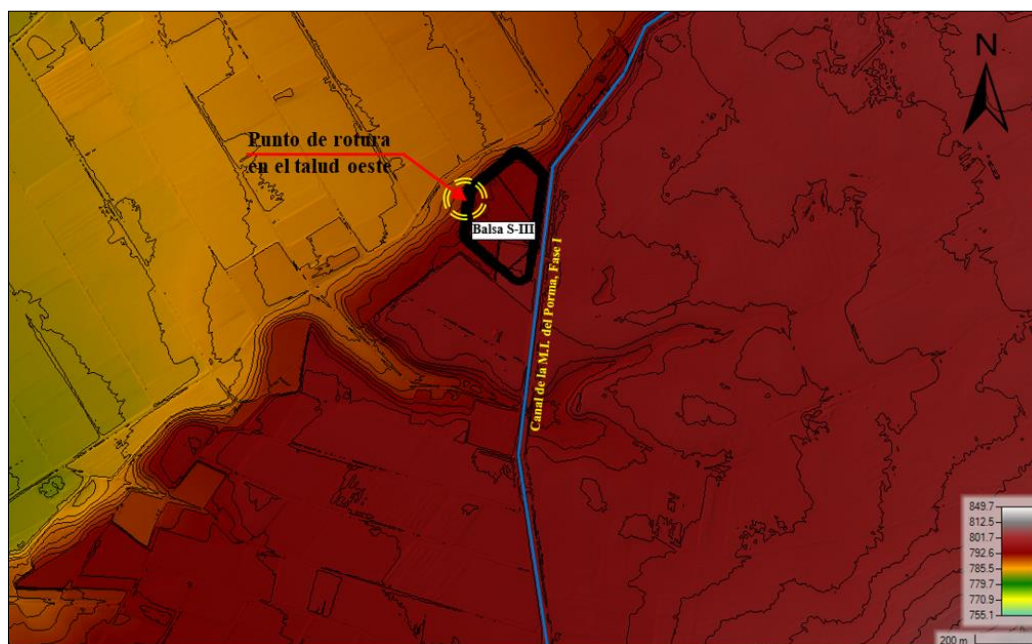
Ilustración 275.- Estudio de rotura de la balsa del S-III. Ubicación del punto de rotura.
