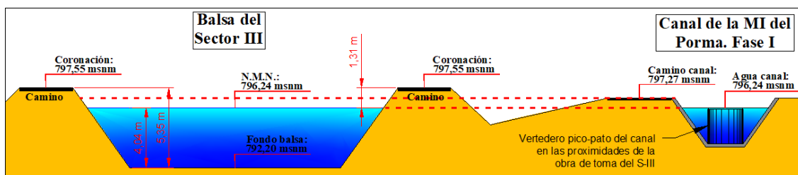
Ilustración 274.- Esquema de cotas de la balsa del S-III y del Canal de la MI del Porma, Fase I.
