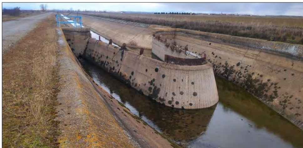
Ilustración 236.- Vertedero pico-pato en la futura obra de toma del sector II.
