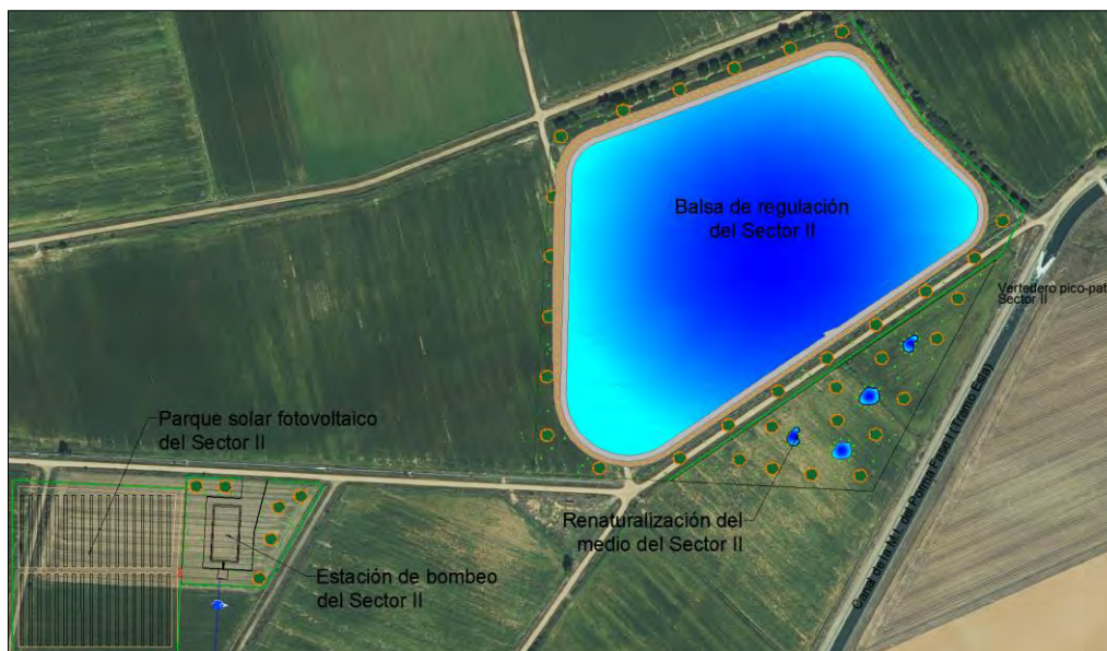
Ilustración 27.- Balsa de regulación del sector II.
