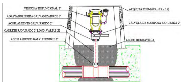
Ilustración 35.- Ejemplo de una ventosa trifuncional instalada en una red de riego.
