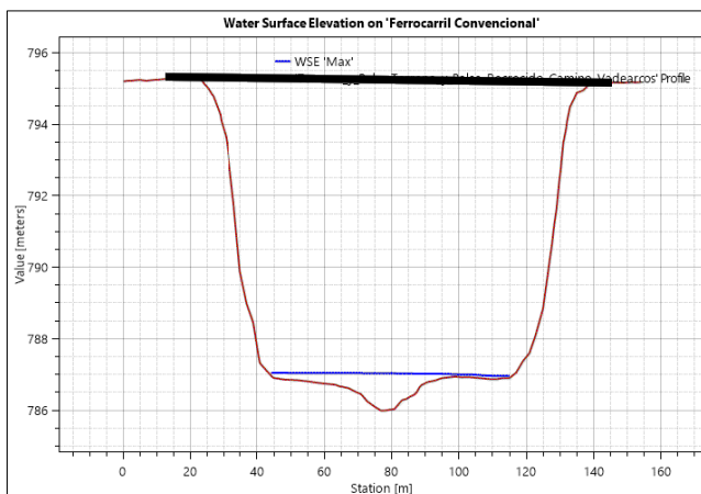
Ilustración 250.- Gráfico de calado en el puente de la línea de FFCC León-Palencia sobre el Arroyo Valdearcos.
