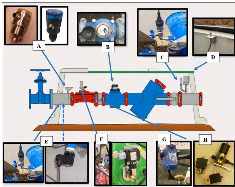
Ilustración 37.- Componentes de un hidrante de riego.
