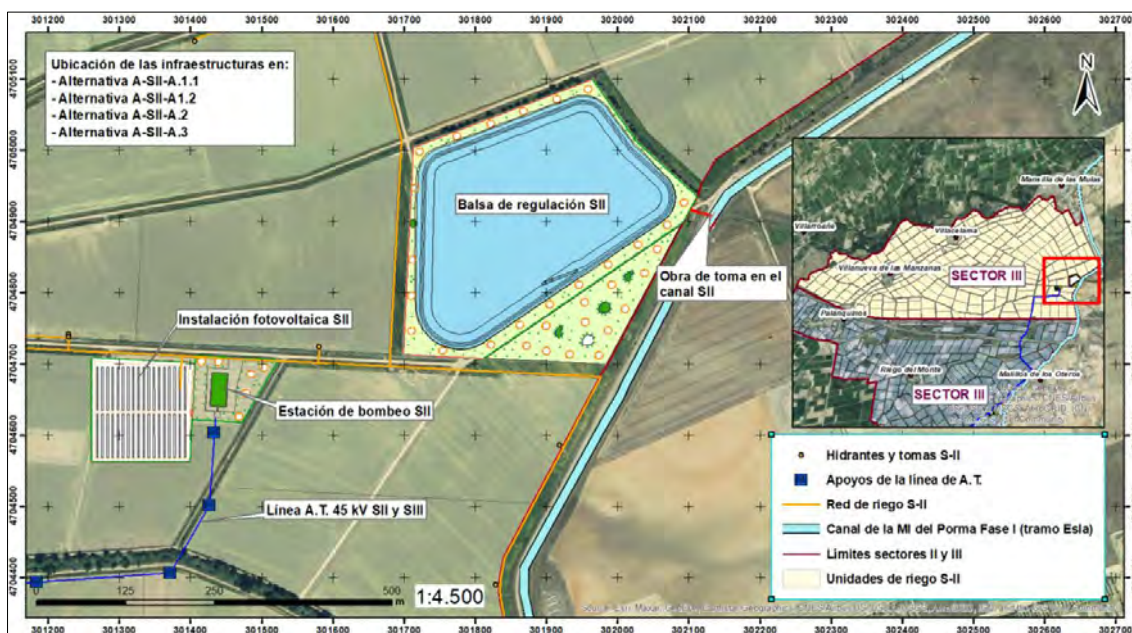
Ilustración 14.- Ubicación de las infraestructuras del S-II en las alternativas A-SII-1.1, A-SII-1.2, A-SII-2 y A-SII-3.
