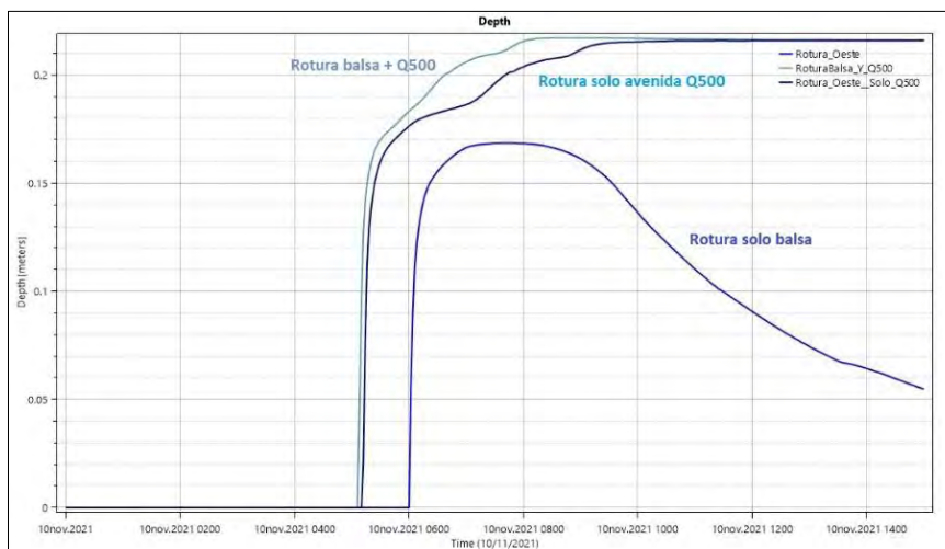
Ilustración 270.- Envoltente de calado en punto de afección a la carretera LE-5506. Escenario de rotura y avenida Q_{500} .
