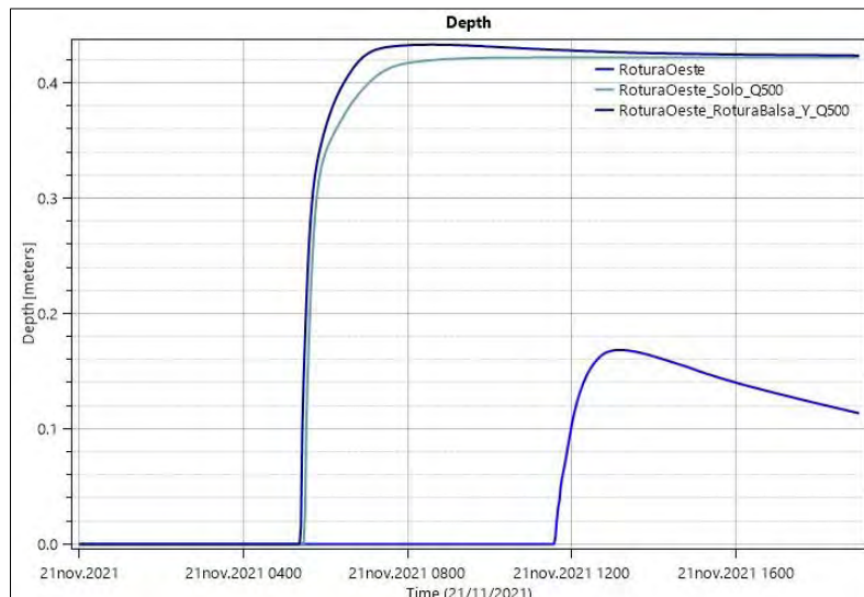
Ilustración 302.- Envolvente de calado en punto de afección del conjunto de tres naves agrícolas en situación rotura S-III más avenida Q500.
