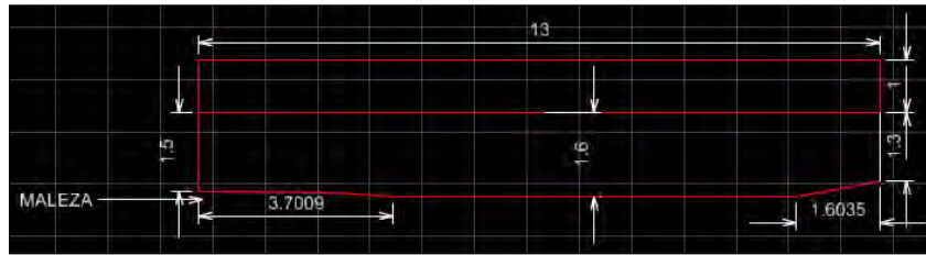
Ilustración 258.- Geometría puente del camino agrícola 2 sobre el Arroyo Valdearcos.
