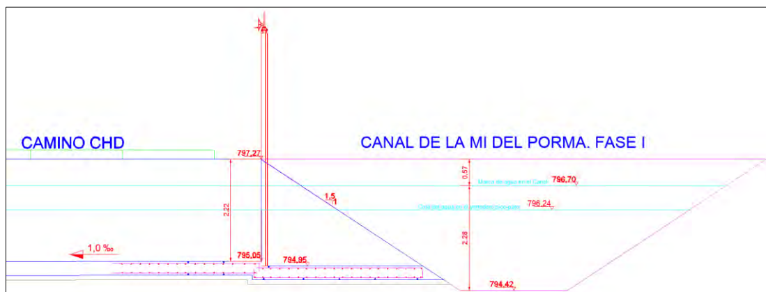
Ilustración 25.- Vista en sección de la compuerta y canal de abastecimiento a balsa del sector III.
