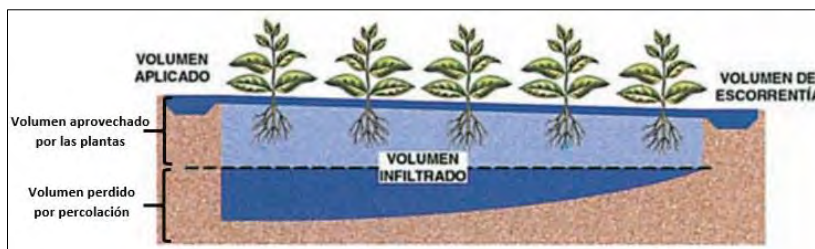
Ilustración 200.- Representación de la pérdida de agua por percolación y por escorrentía en un riego por inundación. Fuente: Manual de riego para agricultores. Sevilla 2010. Junta de Andalucía. Consejería de Agricultura y Pesca.
