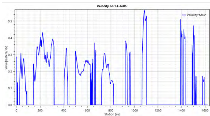
Ilustración 294.- Gráfico de velocidad máxima en la afección n.º 3 sobre la carretera LE-6605.
