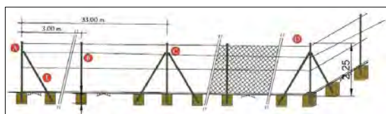
Ilustración 44.- Ejemplo de vallado perimetral de los parques fotovoltaicos.
