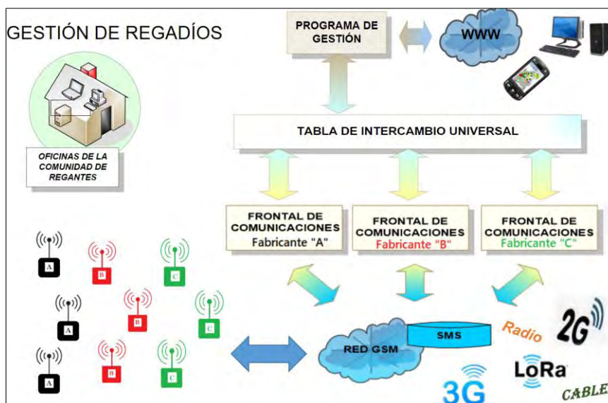
Ilustración 38.- Componentes que forman el entorno el sistema de telecontrol de la red de riego.
