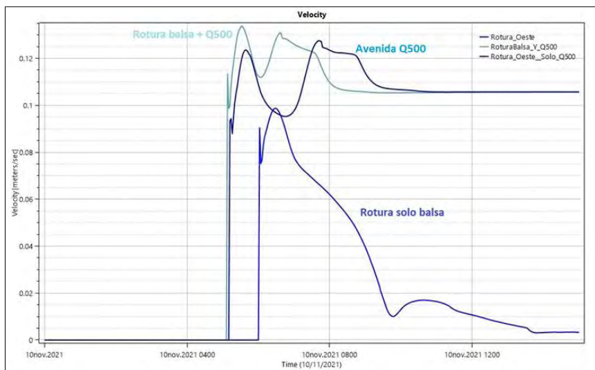
Ilustración 271.- Envolvente de velocidad en punto de afección a la carretera LE-5506. Escenario de rotura y avenida Q500.
