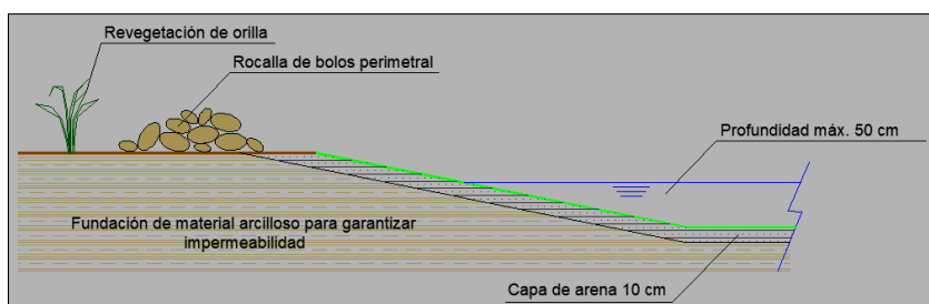
Ilustración 324.- Detalle constructivo del lecho y talud de las charcas.
