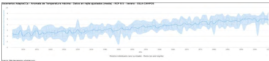
Ilustración 211.- Anomalía de temperatura máxima. Zona agrícola: ESLA-CAMPOS. Escenario 8,5.
