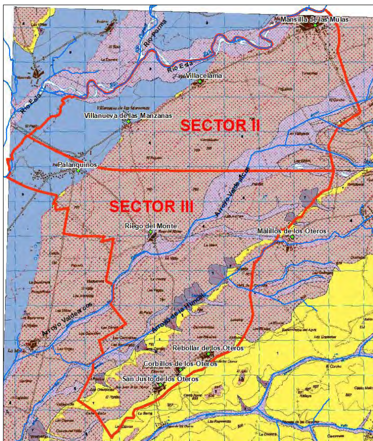
Ilustración 60.- Marco geológico en la ubicación del proyecto de modernización de los Sectores II y III. Fuente: Hoja 195: Mansilla de las Mulas . Escala 1:50.000. Mapa Geológico de España. IGME.
