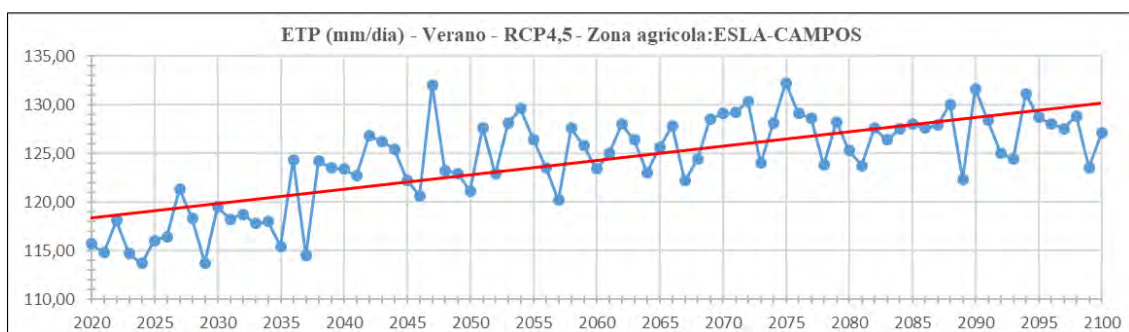
Ilustración 226.- Proyección de la ETP en verano. RCP4,5 entre 2020 y 2100.
