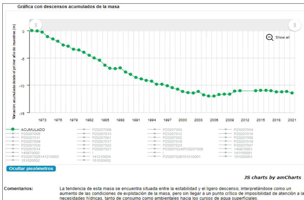
Ilustración 132.- Descensos acumulados de la masa subterránea DU-400008 Terciario y Cuaternario del Esla-Cea. Fuente: Mirame-IDEDuero de Confederación Hidrográfica del Duero.
