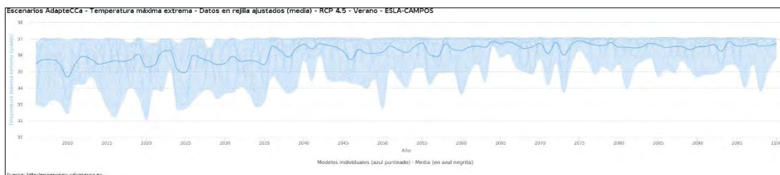
Ilustración 204.- Temperatura máxima extrema. Zona agrícola: ESLA-CAMPOS. Escenario RCP 4,5.
