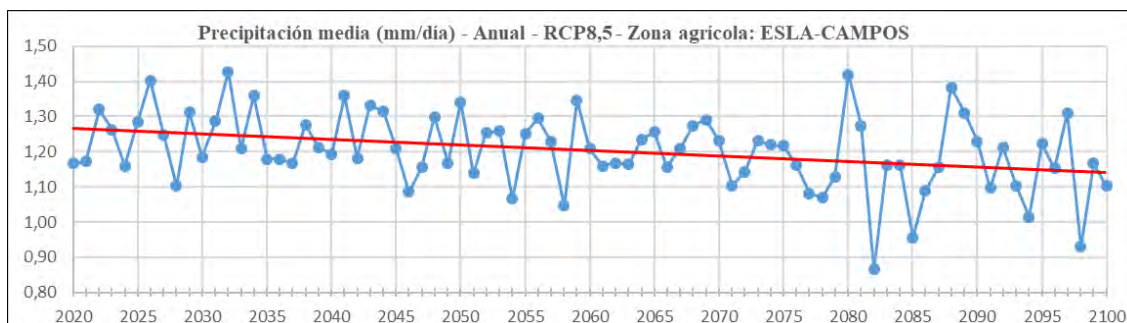
Ilustración 219.- Proyección de la precipitación media diaria. RCP8,5 entre 2020 y 2100.
