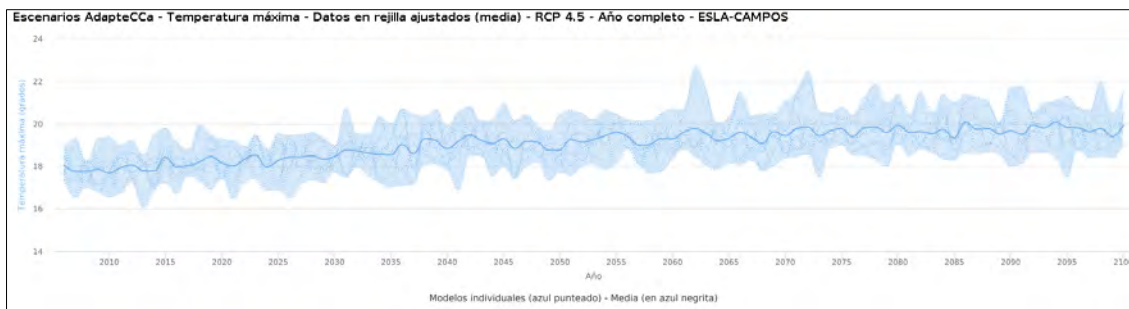
Ilustración 208.- Temperatura máxima media. Zona agrícola: ESLA-CAMPOS. Escenario RCP 4,5.
