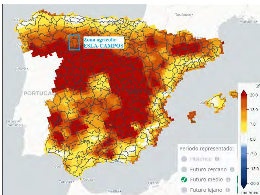
Ilustración 228.- Proyección de la evapotranspiración potencial (ETP) en un futuro medio. Verano escenario RCP8,5.
