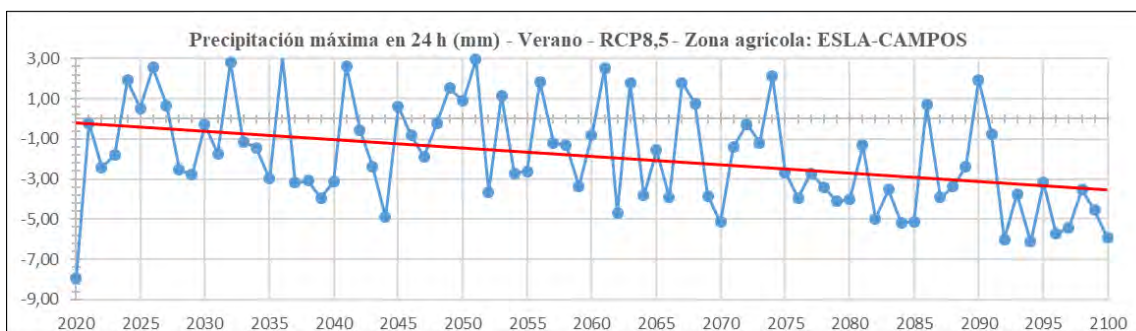
Ilustración 225.- Proyección de las precipitaciones máximas en 24 horas en verano. RCP8,5 entre 2020 y 2100.
