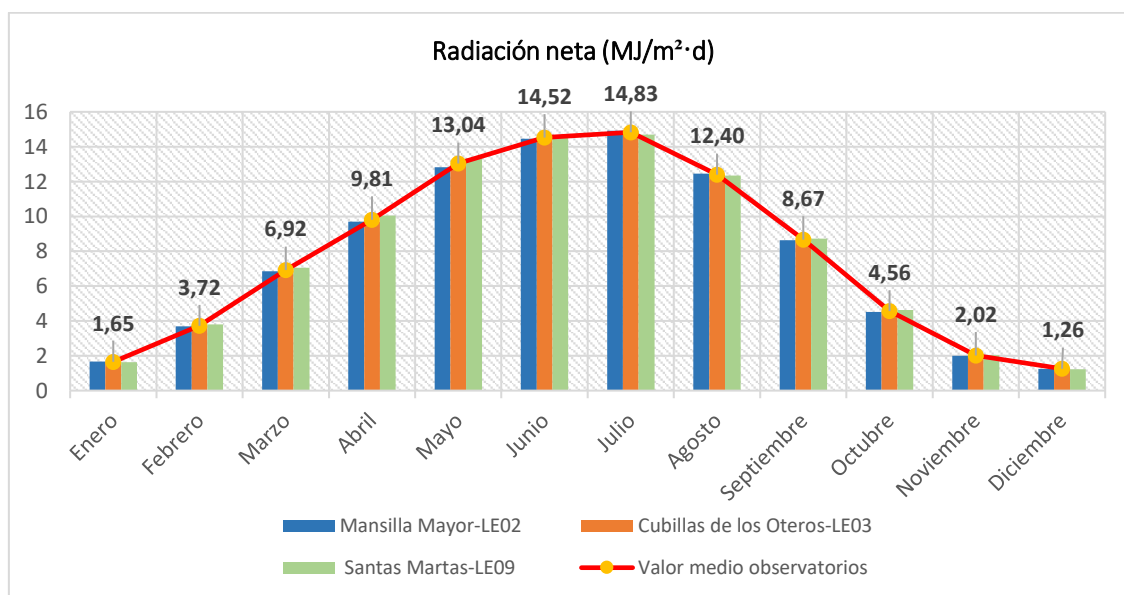
Gráfico 6.- Radiación neta media mensual en la zona de estudio. Fuente: elaboración propia. Base de datos meteorológicos red INFORIEGO y red AEMET.
