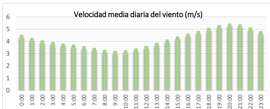
Gráfico 5.- Perfil medio diario de la velocidad del viento en la zona del proyecto. Fuente: Atlas Eólico Ibérico del IDAE.
