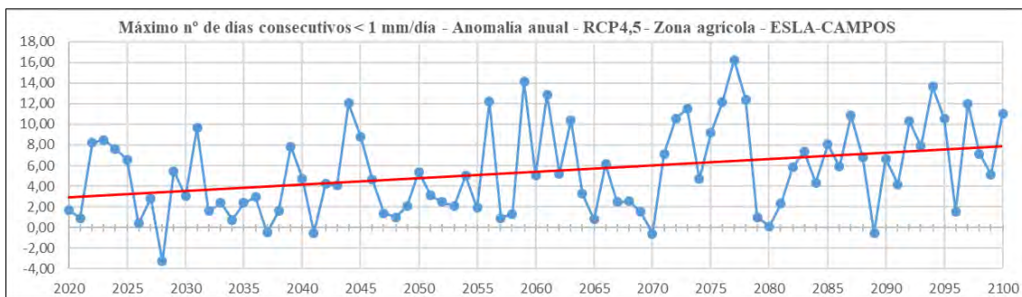
Ilustración 220.- Proyección del nº de días consecutivos con precipitación < 1 mm/día. RCP4,5 entre 2020 y 2100.
