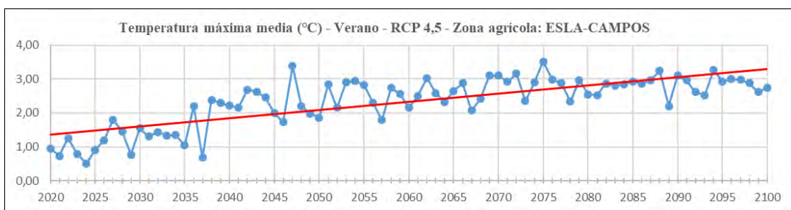
Ilustración 212.- Proyección de la temperatura máxima media en verano RCP4,5 entre 2020 y 2100.
