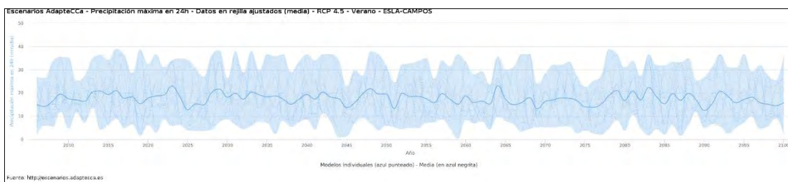
Ilustración 222.- Precipitación máxima en 24 h. Zona agrícola: ESLA-CAMPOS. Verano. Escenario RCP 4,5.
