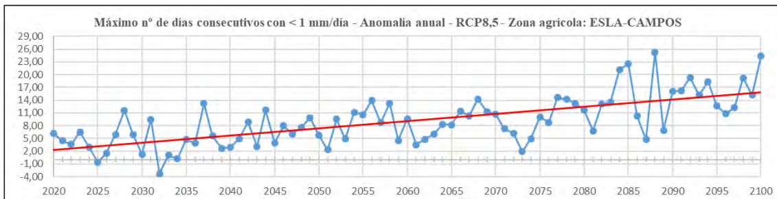
Ilustración 221.- Proyección del nº de días consecutivos con precipitación < 1 mm/día. RCP8,5 entre 2020 y 2100.
