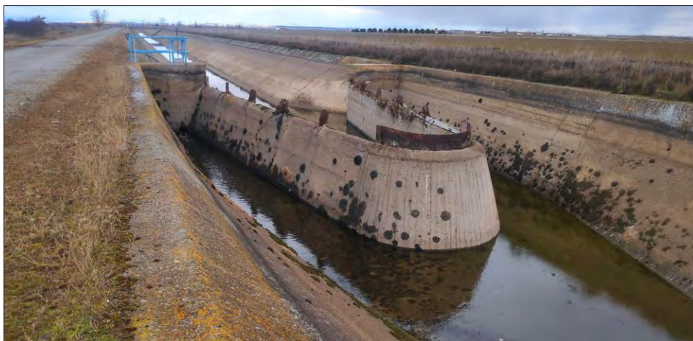
Ilustración 20.- Vertedero pico-pato del sector II.
