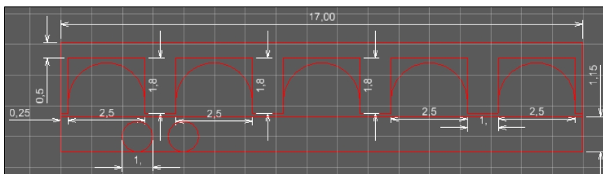
Ilustración 287.- Geometría del puente de la carretera LE-512 sobre el Arroyo Valdearcos.
