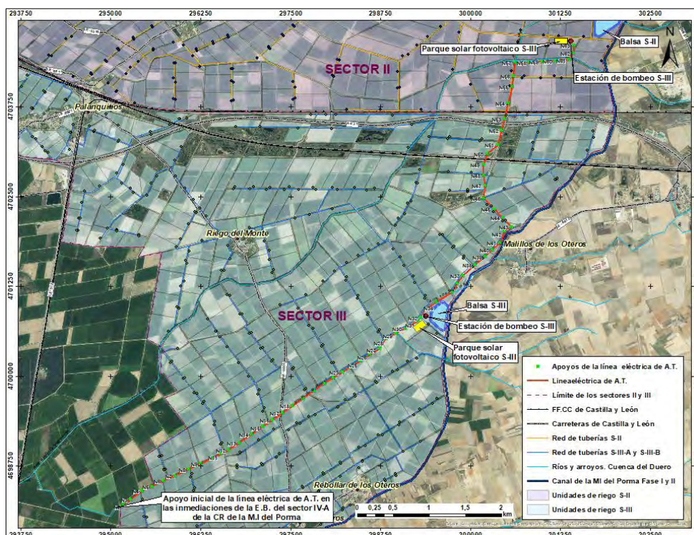
Ilustración 42.- Trazo de la línea eléctrica de Alta Tensión. Abastecimiento de las E.B de los sectores II y III.
