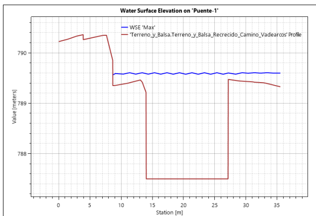
Ilustración 256.- Gráfico de calado en el puente del camino agrícola 1 sobre el Arroyo Valdearcos.
