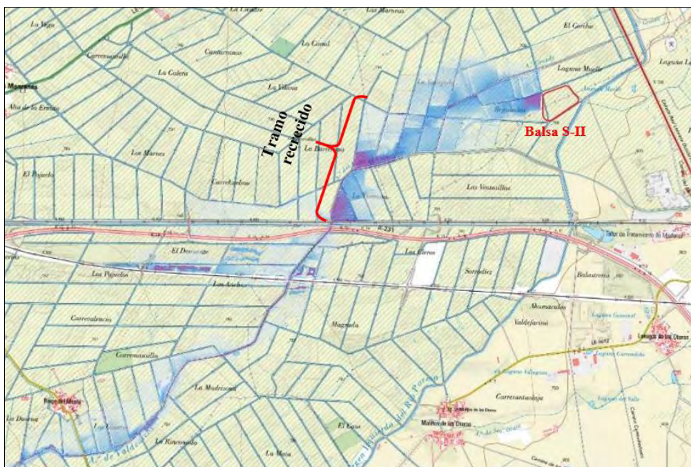
Ilustración 240.- Trayectoria de la onda de avenida en la rotura de la balsa S-II con el recercado del camino.
