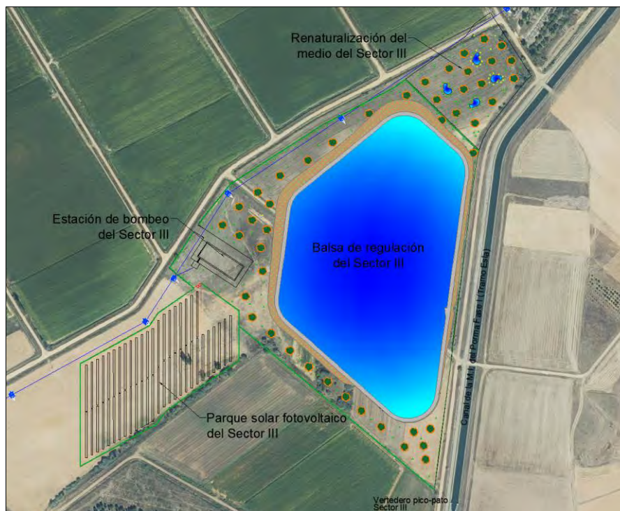
Ilustración 28.- Balsa de regulación del sector III.
