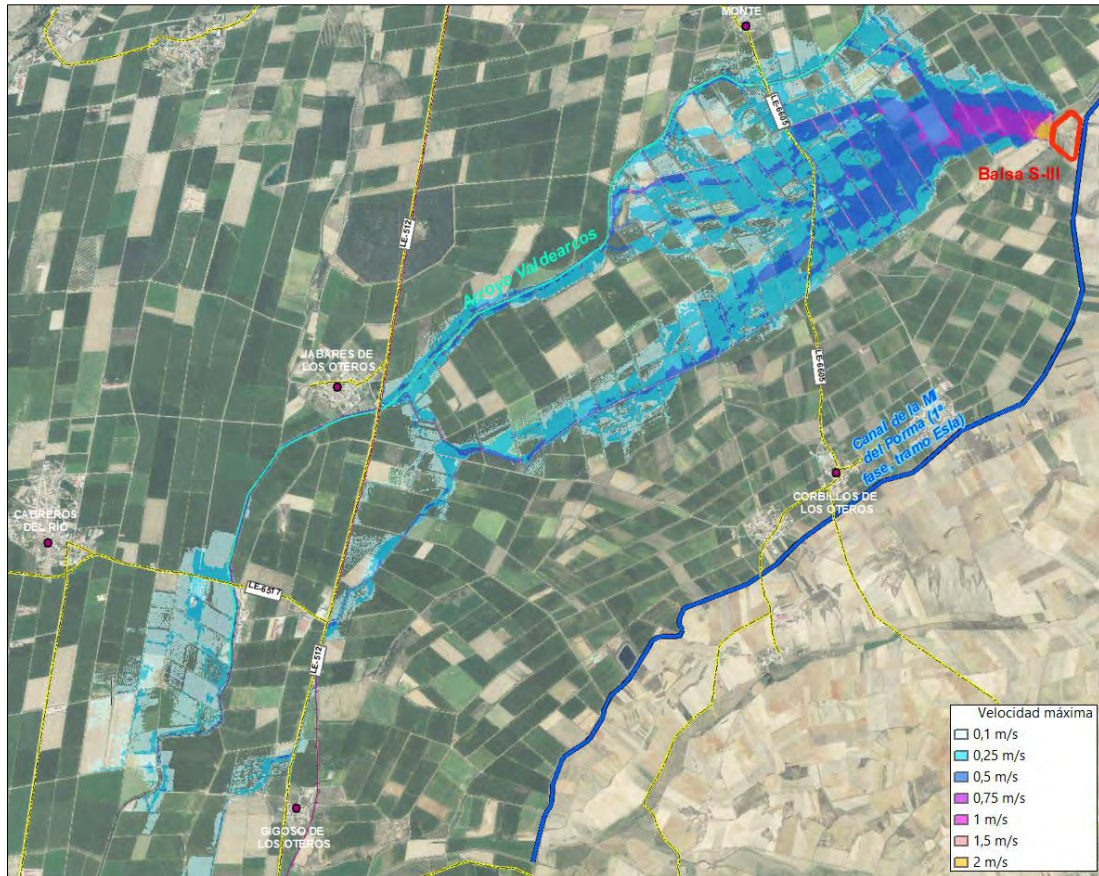
Ilustración 282.- Envolve de velocidad máxima rotura balsa sector III.
