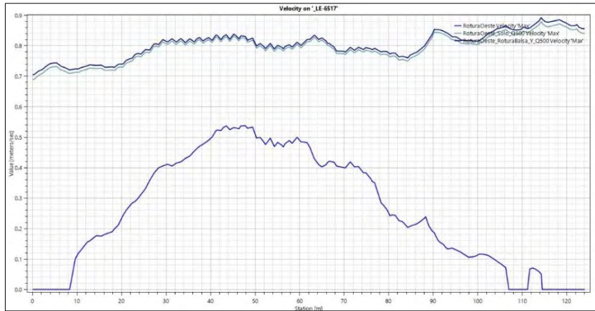
Ilustración 301.- Velocidad en punto de afección de la carretera LE-6517 en situación rotura S-III más avenida Q500.
