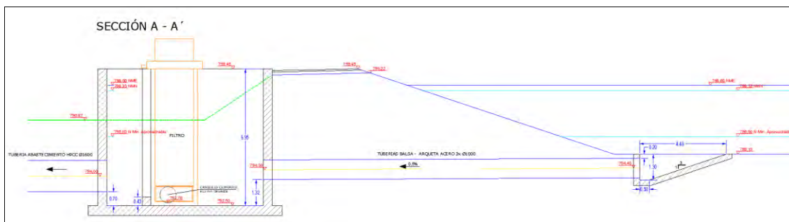
Ilustración 31.- Vista en sección de la toma en balsa, tuberías de acero y arqueta de filtros del sector II.
