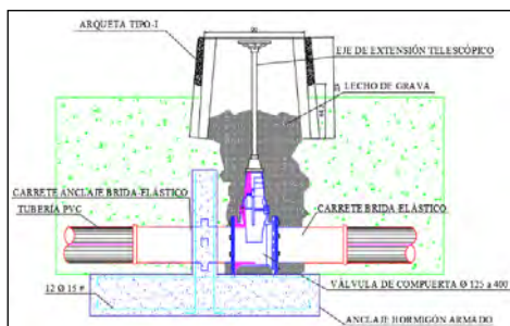
Ilustración 34.- Ejemplo de una válvula de corte de la red de tuberías.
