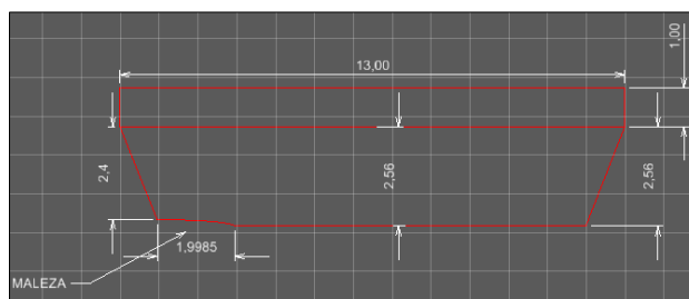
Ilustración 264.- Geometría del puente de la carretera LE-6605 sobre el Arroyo Valdearcos.
