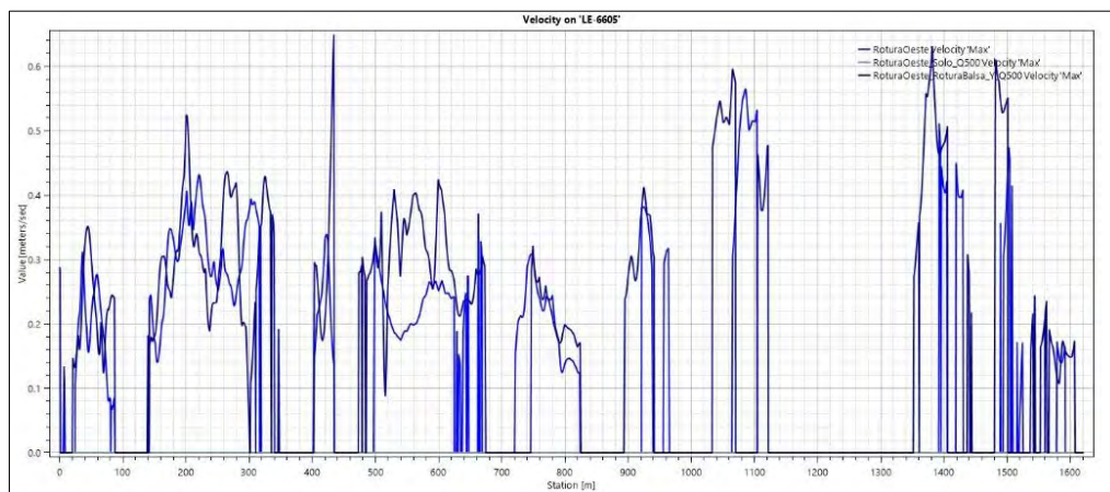
Ilustración 299.- Velocidad en punto de afección de la carretera LE-6605 en situación rotura S-III más avenida Q500.
