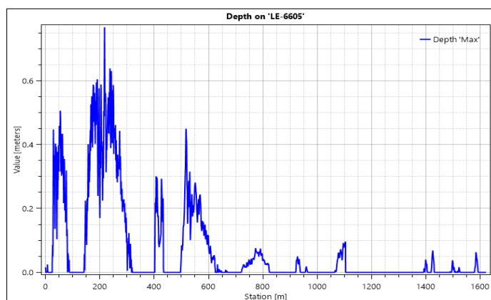
Ilustración 293.- Gráfico de calado máximo en la afección n.º 3 sobre la carretera LE-6605.
