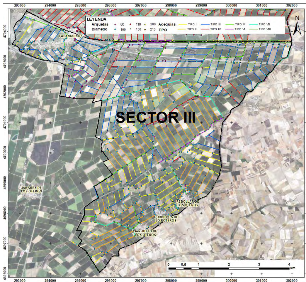
Ilustración 48.- Traza de la red de acequias a retirar en el sector III.
