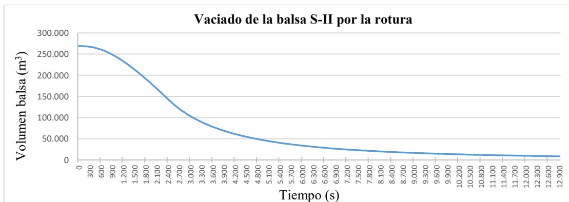
Ilustración 242.- Curva de vaciado en la simulación de la rotura de la balsa del S-II.
