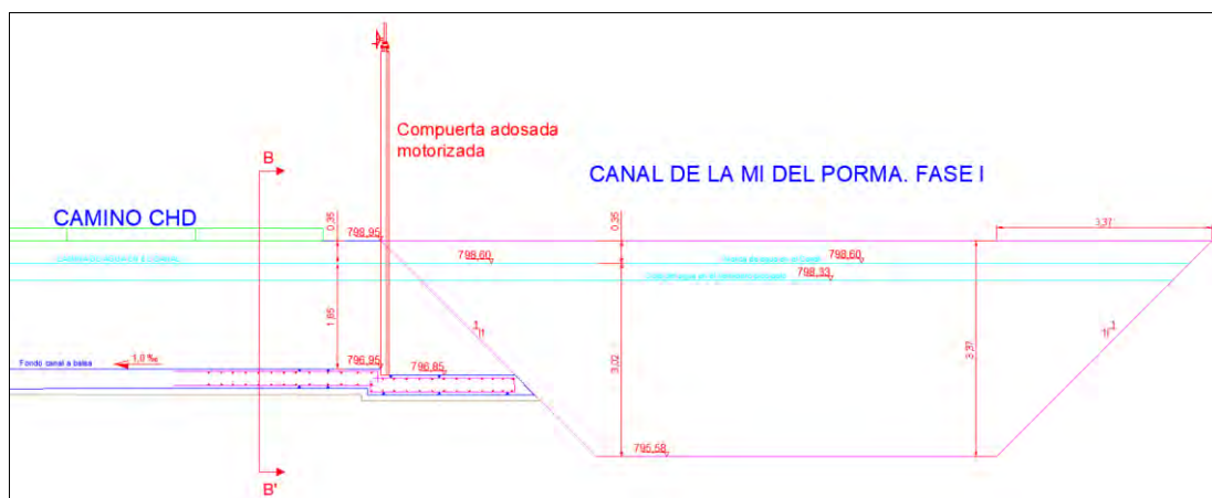
Ilustración 22.- Vista en sección de la compuerta y canal de abastecimiento a balsa del sector II.
