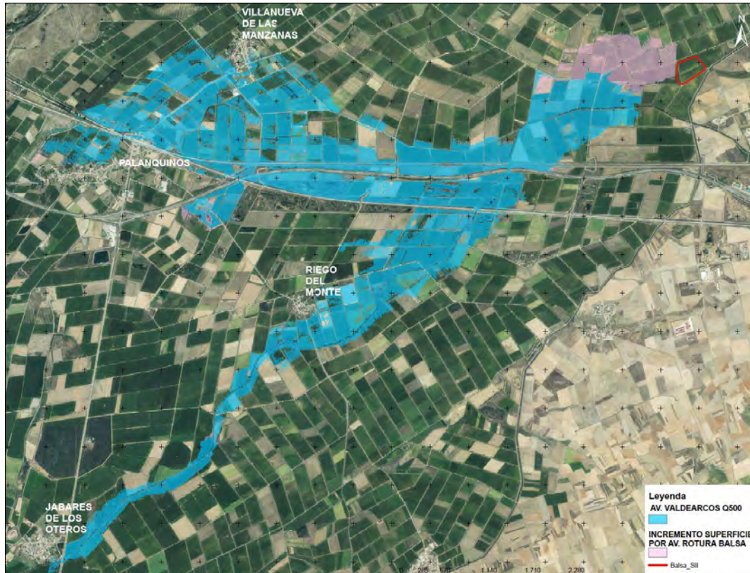
Ilustración 269.- Incremento de superficie planteando la rotura de la balsa S-II y la avenida del Arroyo Valdearcos para Q_{500} .
