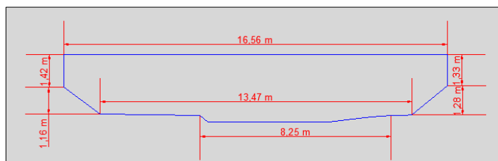
Ilustración 289.- Geometría del puente de la carretera LE-6517 sobre el Arroyo Valdearcos.
