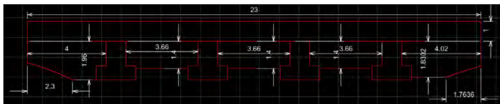
Ilustración 249.- Geometría del puente de la línea de FFCC convencional León-Palencia sobre el Arroyo Valdearcos.
