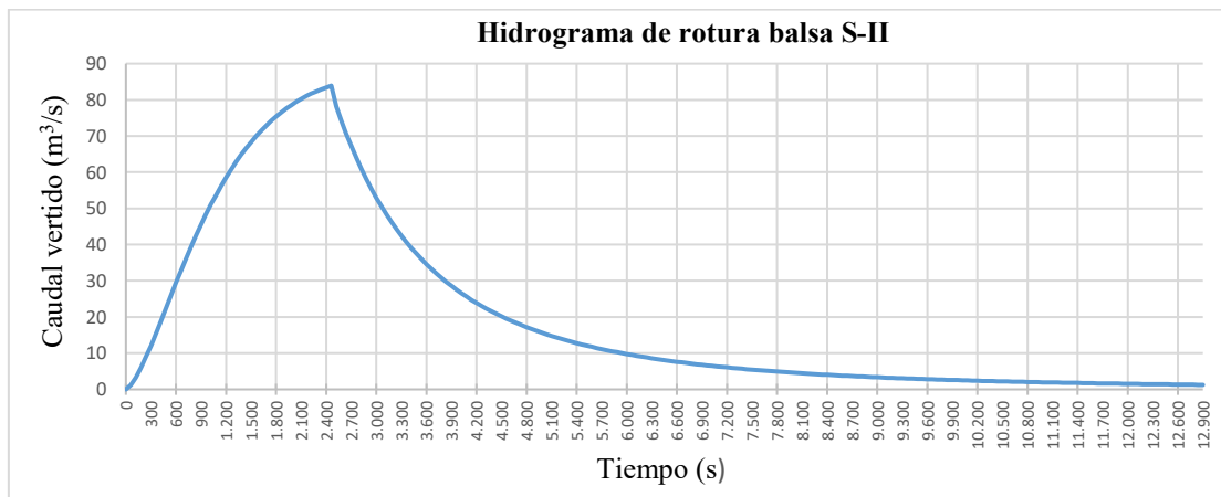
Ilustración 241.- Hidrograma de rotura para la simulación de la balsa del S-II.
