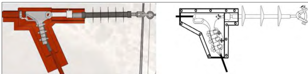
Ilustración 320.- Grapas de amarre, forro tipo FOGR.
