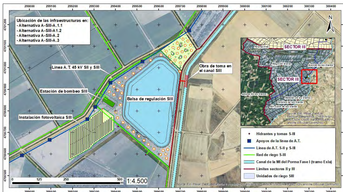
Ilustración 15.- Ubicación de las infraestructuras del S-III en las alternativas A-SIII-1.1, A-SIII-1.2, A-SIII-2 y A-SIII-3.
