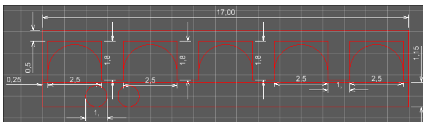
Ilustración 266.- Geometría del puente de la carretera LE-512 sobre el Arroyo Valdearcos.
