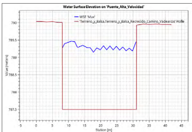
Ilustración 262.- Gráfico de calado en el puente de la línea de FFCC de alta velocidad Venta de Baños-León sobre el Arroyo Valdearcos.
