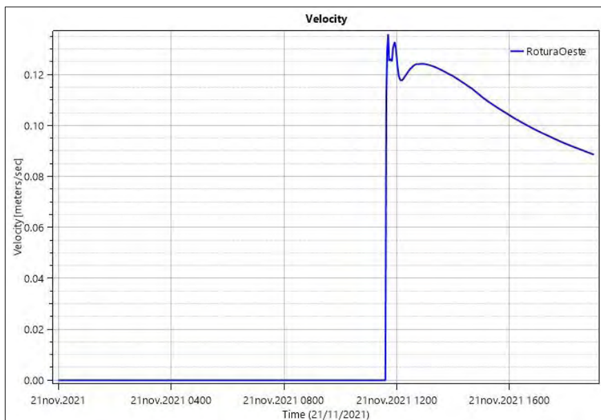
Ilustración 292.- Envolve de velocidad en el punto de la afección n.º 5 conjunto de tres naves agrícolas.
