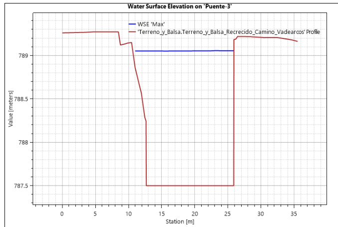
Ilustración 259.- Gráfico de calado en el puente del camino agrícola 2 sobre el Arroyo Valdearcos.
