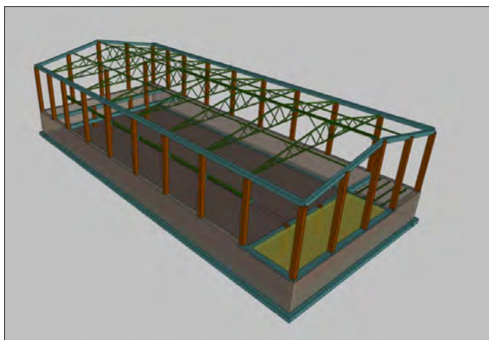
Ilustración 40.- Imagen 3D de la estructura de la nave para la estación de bombeo del sector II.
