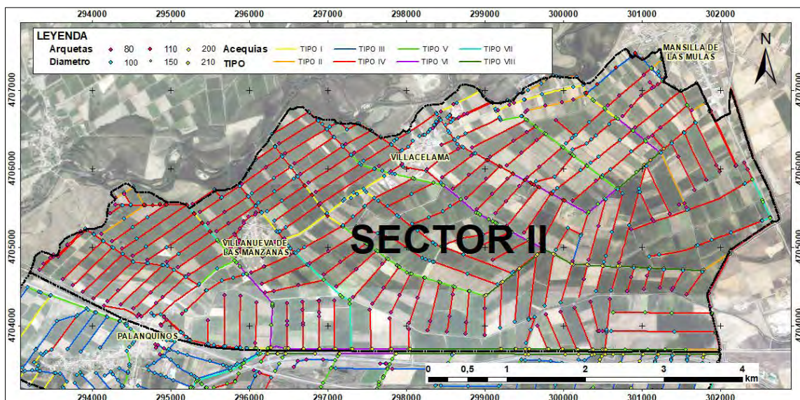
Ilustración 47.- Trazo de la red de acequias a retirar en el sector II.
