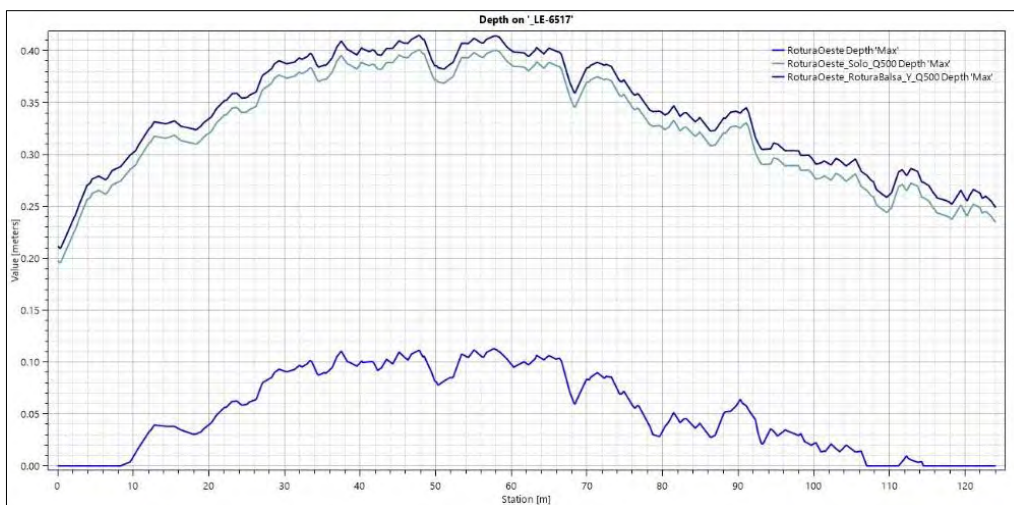
Ilustración 298.- Calado en punto de afección de la carretera LE-6605 en situación rotura S-III más avenida Q500.
