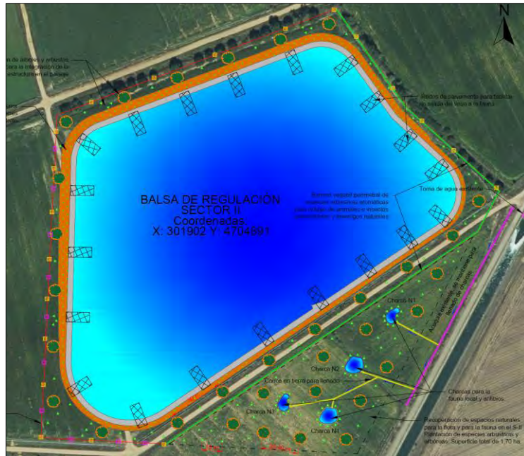
Ilustración 336.- Ubicación de la barrera vegetal de especies aromáticas y plantación para mitigar el impacto visual, balsa del S-II.
