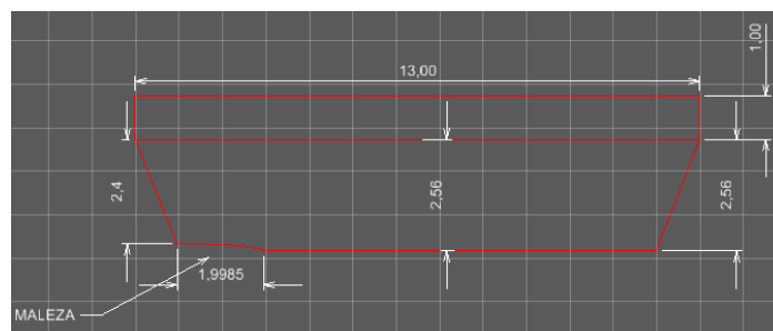
Ilustración 285.- Geometría del puente de la carretera LE-6605 sobre el Arroyo Valdearcos.
