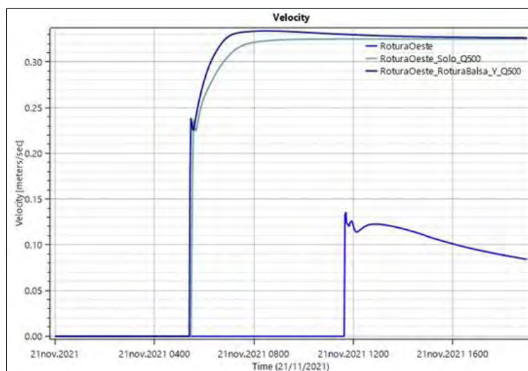
Ilustración 303.- Envolvente de velocidad en punto de afección del conjunto de tres naves agrícolas en situación rotura S-III más avenida Q500.
