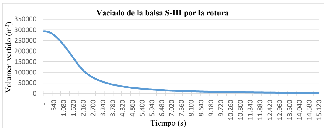
Ilustración 278.- Curva de vaciado en la simulación de la rotura de la balsa del S-III.
