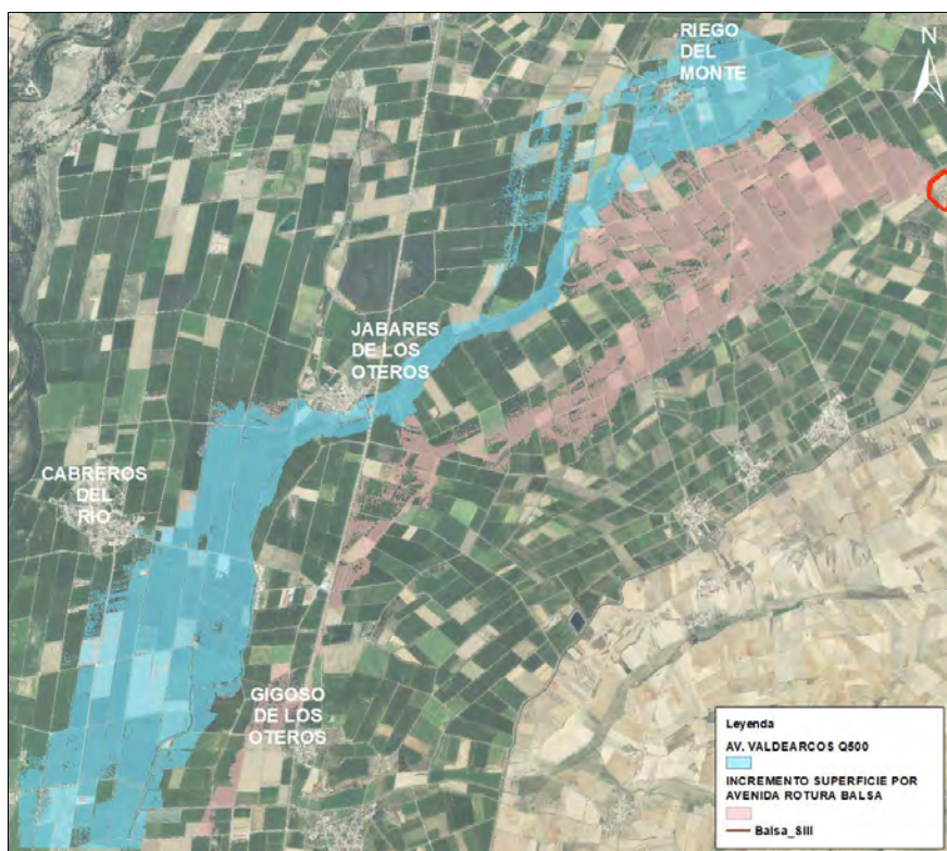
Ilustración 297.- Incremento de superficie planteando la rotura de la balsa S-III y la avenida del Arroyo Valdearcos para Q500.
