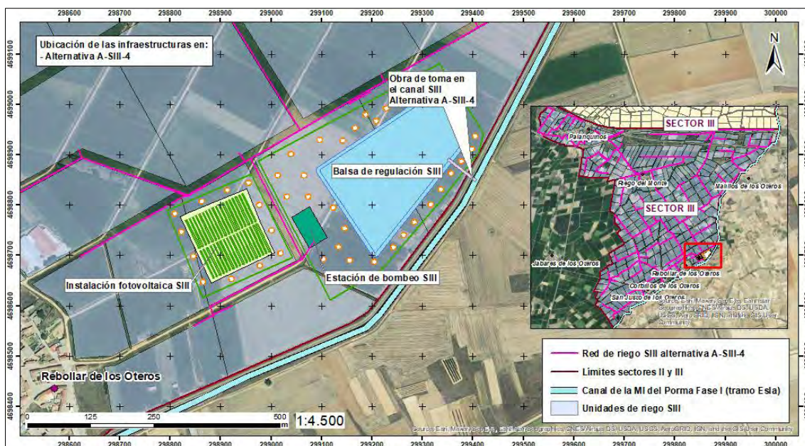
Ilustración 16.- Ubicación de las infraestructuras del S-III en las alternativas A-SIII-1.1, A-SIII-4.
