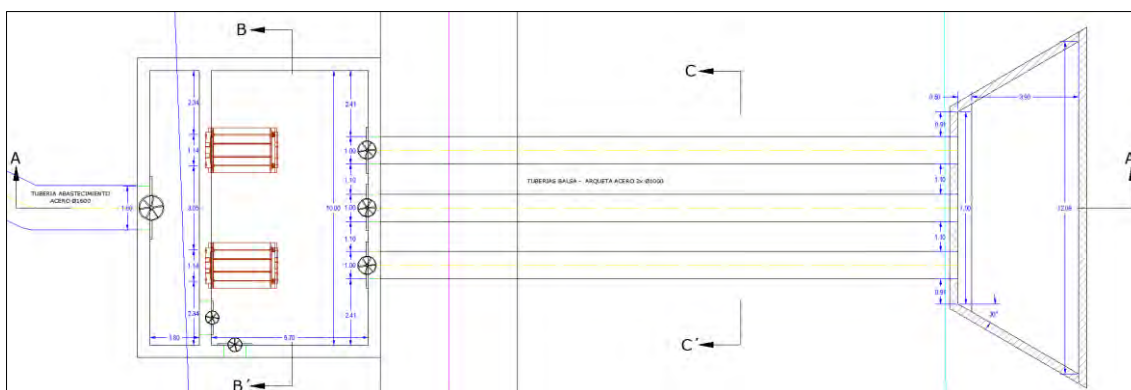
Ilustración 32.- Vista en planta de la toma en balsa y arqueta de filtros del sector III.
