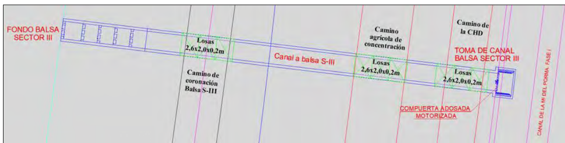
Ilustración 26.- Vista en planta del canal de abastecimiento a balsa y obra de toma del sector III.
