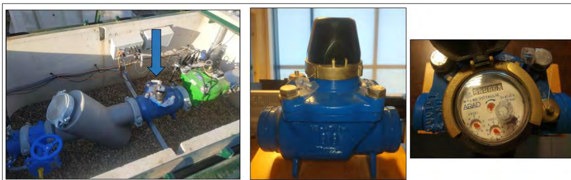
Ilustración 307.- Ejemplo de caudalímetro instalado en un hidrante.
