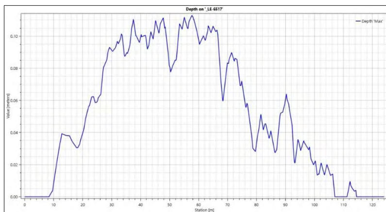
Ilustración 295.- Gráfico de calado máximo en la afección n.º 3 sobre la carretera LE-6617.
