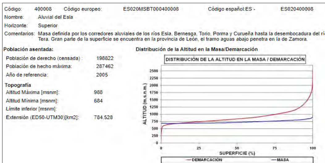
Ilustración 126.- Ficha técnica de la masa subterránea del horizonte superior DU 400008 - Aluvial del Esla . Fuente: Mirame-IDEDuero de Confederación Hidrográfica del Duero.
