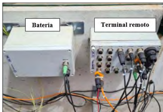
Ilustración 39.- Ejemplo de un terminal remoto instalado en un hidrante.
