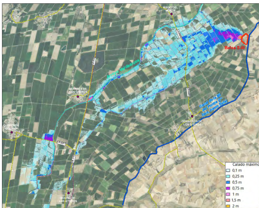
Ilustración 281.- Envoltente de calado máximo rotura balsa sector III.
