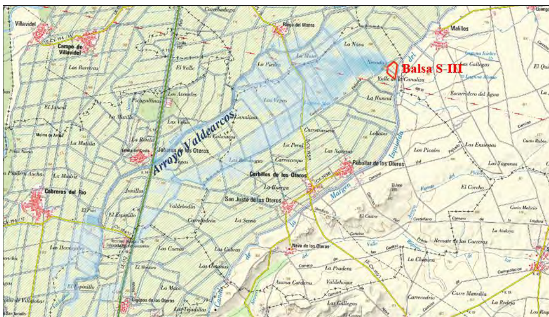
Ilustración 276.- Ubicación de la balsa del sector II respecto de la onda de avenida generada por la rotura.
