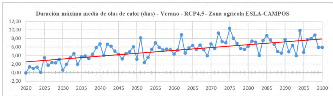
Ilustración 216.- Proyección de la duración de olas de calor media en verano RCP4,5 entre 2020 y 2100. Fuente: Visor de Escenarios de Cambio Climático. escenarios.AdapteCCA.es
