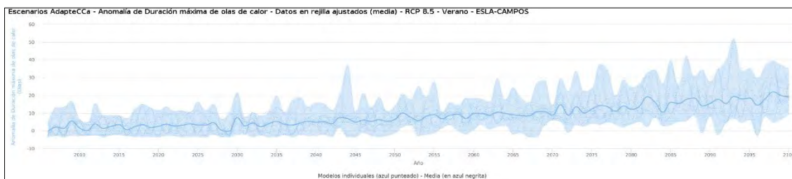
Ilustración 215.- Duración de olas de calor. Zona agrícola: ESLA-CAMPOS. Verano. Escenario RCP 8,5. Fuente: Visor de Escenarios de Cambio Climático. escenarios.AdapteCCA.es
