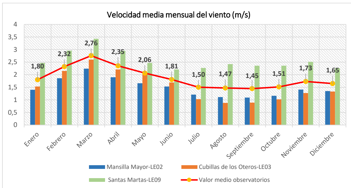
Gráfico 4.- Velocidad media mensual del viento en la zona de estudio. Fuente: elaboración propia. Base de datos meteorológicos red INFORIEGO y red AEMET.
