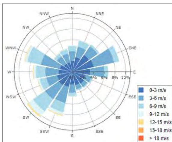
Ilustración 57.- Rosa de los vientos para la ubicación central de la zona del proyecto. Fuente: Atlas Eólico Ibérico del IDAE.
