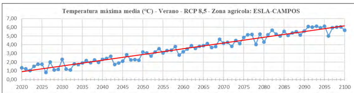
Ilustración 213.- Proyección de la temperatura máxima media en verano RCP8,5 entre 2020 y 2100.
