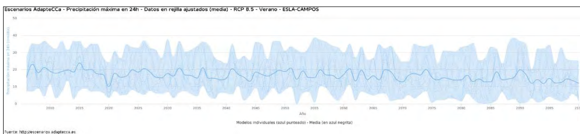
Ilustración 223.- Precipitación máxima en 24 h. Zona agrícola: ESLA-CAMPOS. Verano. Escenario RCP 8,5.
