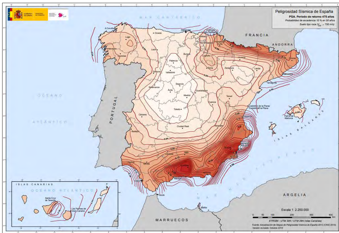
Ilustración 231.- Mapa de peligrosidad Sísmica de España 2015 (en valores de aceleración). Fuente: Mapas de sismicidad y peligrosidad. IGN. ETRS89 – UTM 30N / UTM 28N (Islas Canarias).
