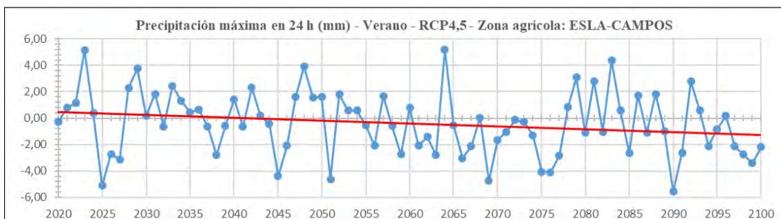
Ilustración 224.- Proyección de las precipitaciones máximas en 24 horas en verano. RCP4,5 entre 2020 y 2100.
