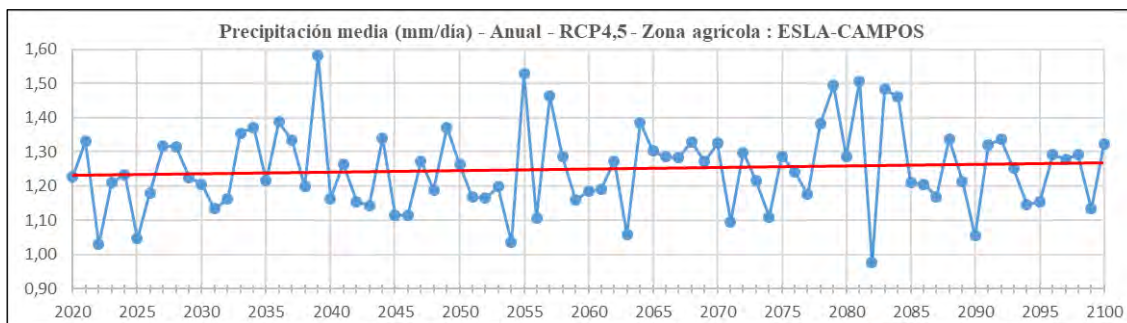
Ilustración 218.- Proyección de la precipitación media diaria. RCP4,5 entre 2020 y 2100.
