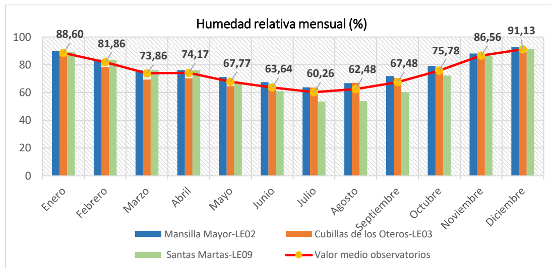
Gráfico 2.- Humedad relativa media mensual en la zona de estudio. Fuente: elaboración propia. Base de datos meteorológicos red INFORIEGO y red AEMET.
