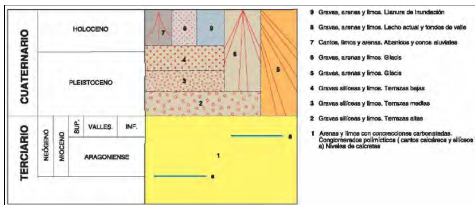
Ilustración 61.- Leyenda del marco geológico de la Hoja 195: Mansilla de las Mulas . Fuente: Hoja 195: Mansilla de las Mulas . Escala 1:50.000. Mapa Geológico de España. IGME.
