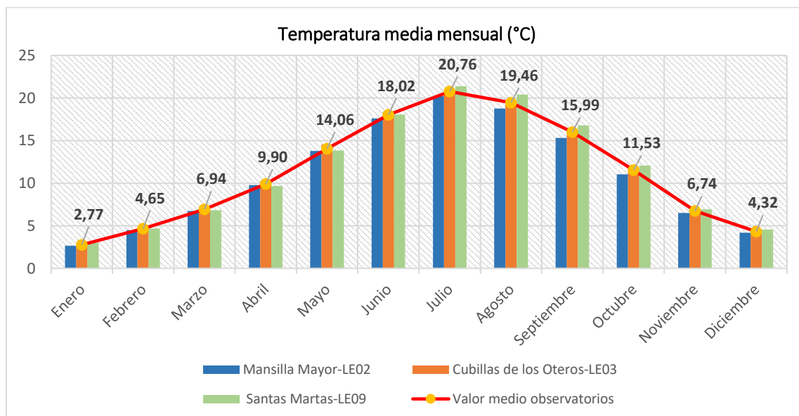
Gráfico 1.- Temperatura media mensual en la zona de estudio. Fuente: elaboración propia. Base de datos meteorológicos red INFORIEGO y red AEMET.
