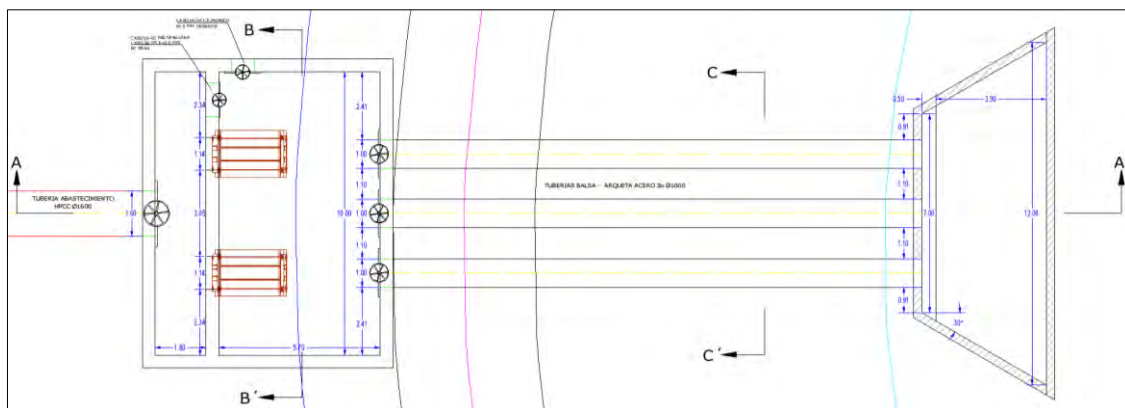
Ilustración 29.- Vista en planta de la toma en balsa y arqueta de filtros del sector II.
