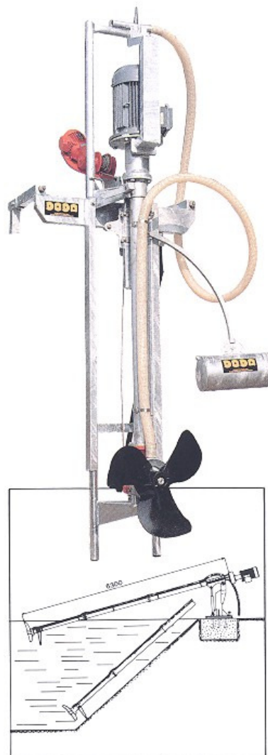
Agitador de paletas (Doda)
