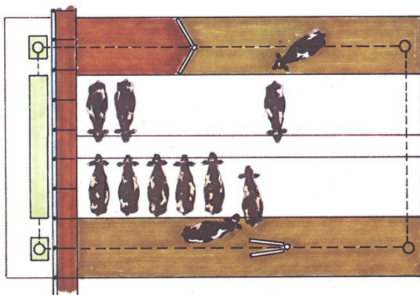
Sistema de limpieza por paletas y cable en estabulación libre (Alfa-Laval)
