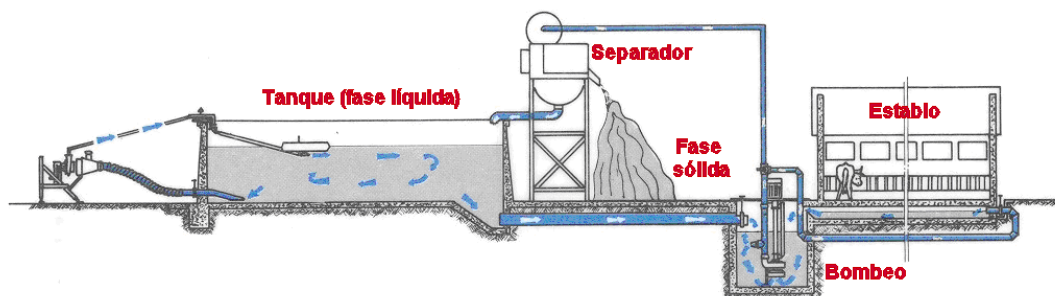
Instalación para la gestión del estiércol con recirculación y separación sólido-líquido (Doda)
