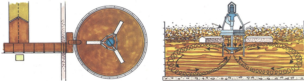
Bomba trituradora vertical (Doda)
