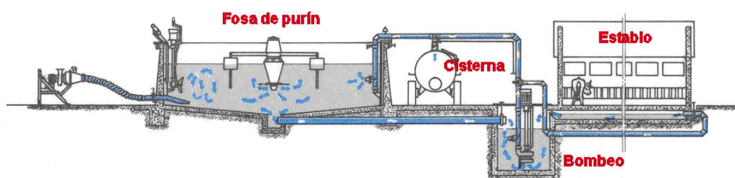
Instalación para la gestión del estiércol con recirculación y separación sólido-líquido (Doda)
