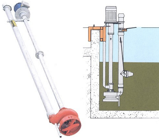
Bomba trituradora vertical (Doda)
