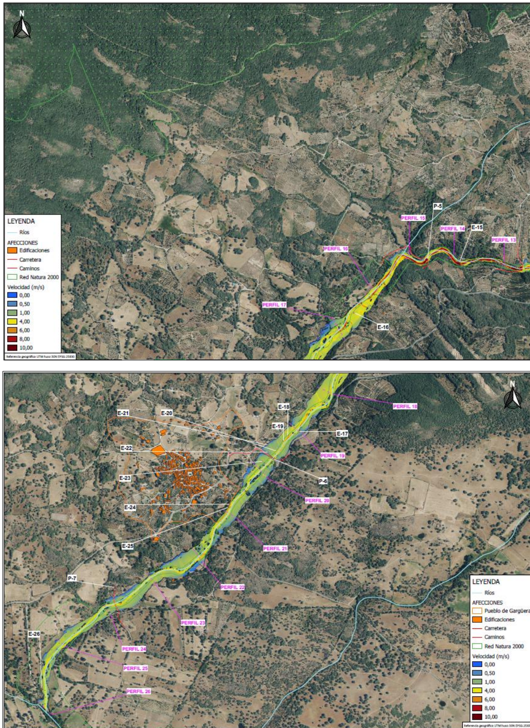
Ilustración 67. Velocidades máximas Balsa 1
