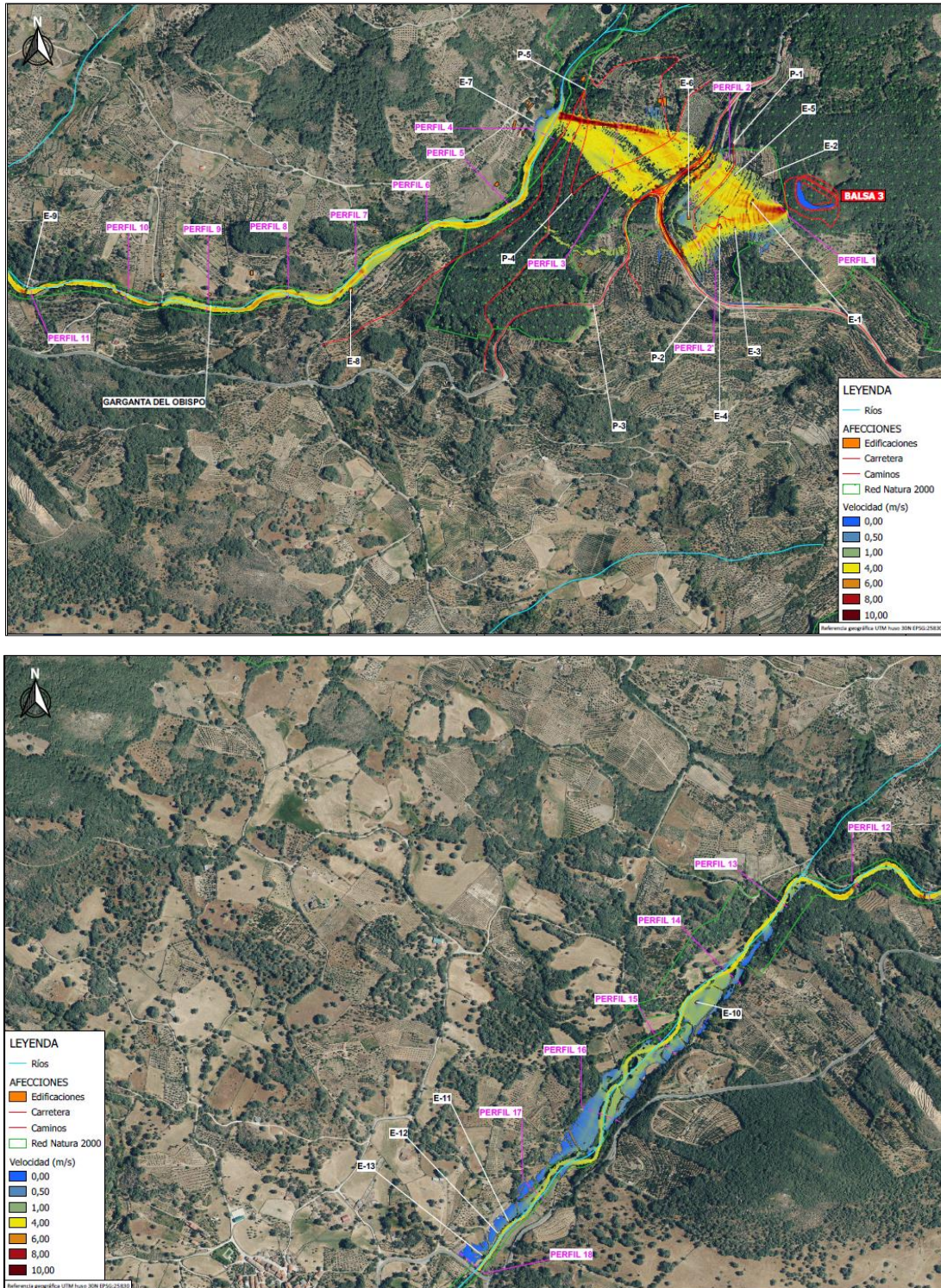
Ilustración 71. Velocidades máximas escenario H2 – suroeste
