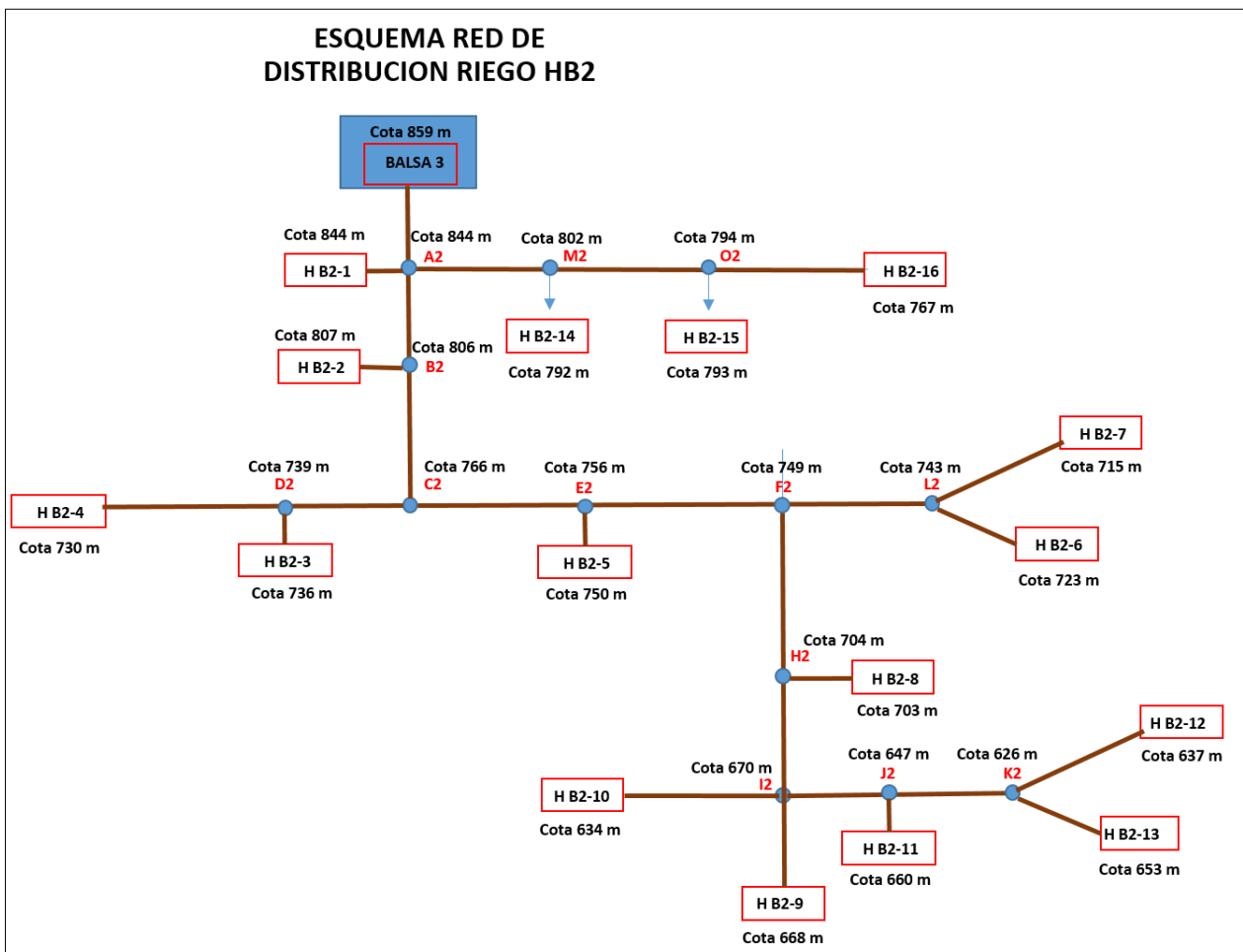
Esquema 8: Esquema Riego HB2
