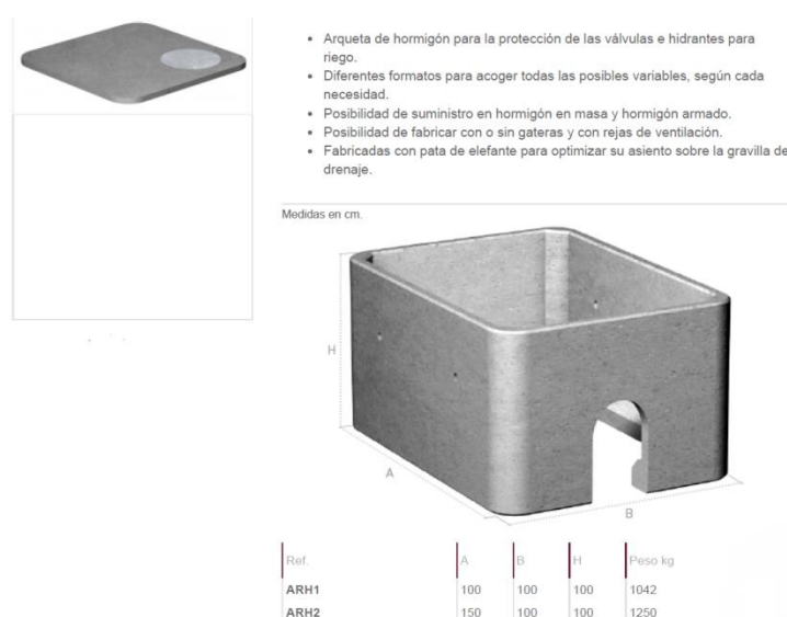
Ilustración 5. Arqueta tipo toma cauce
