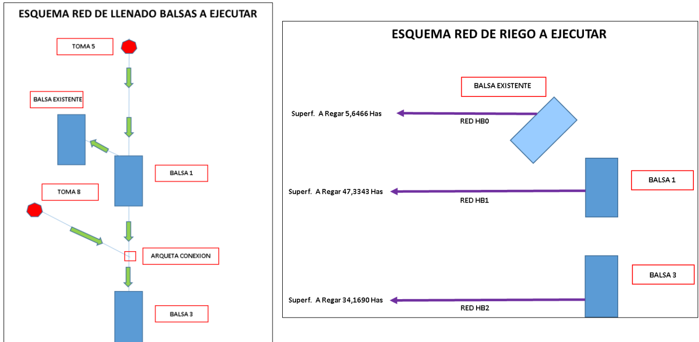
Ilustración 44. Esquema general red.
