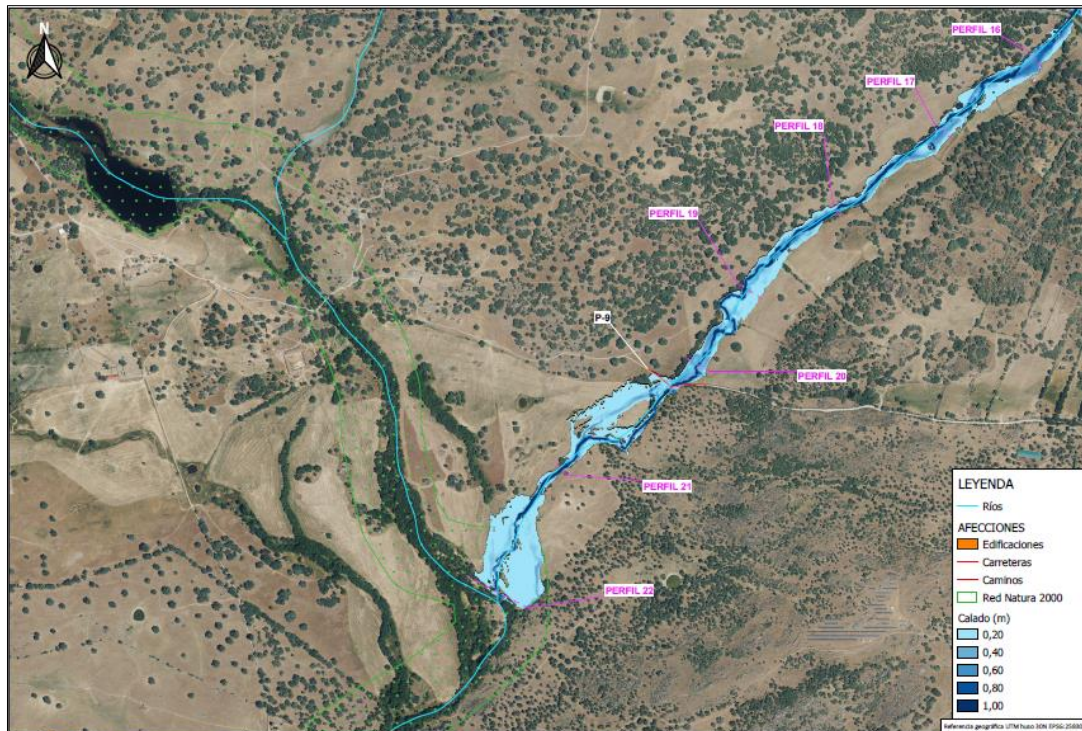
Ilustración 68. Calado máximo escenario H2 – sureste
