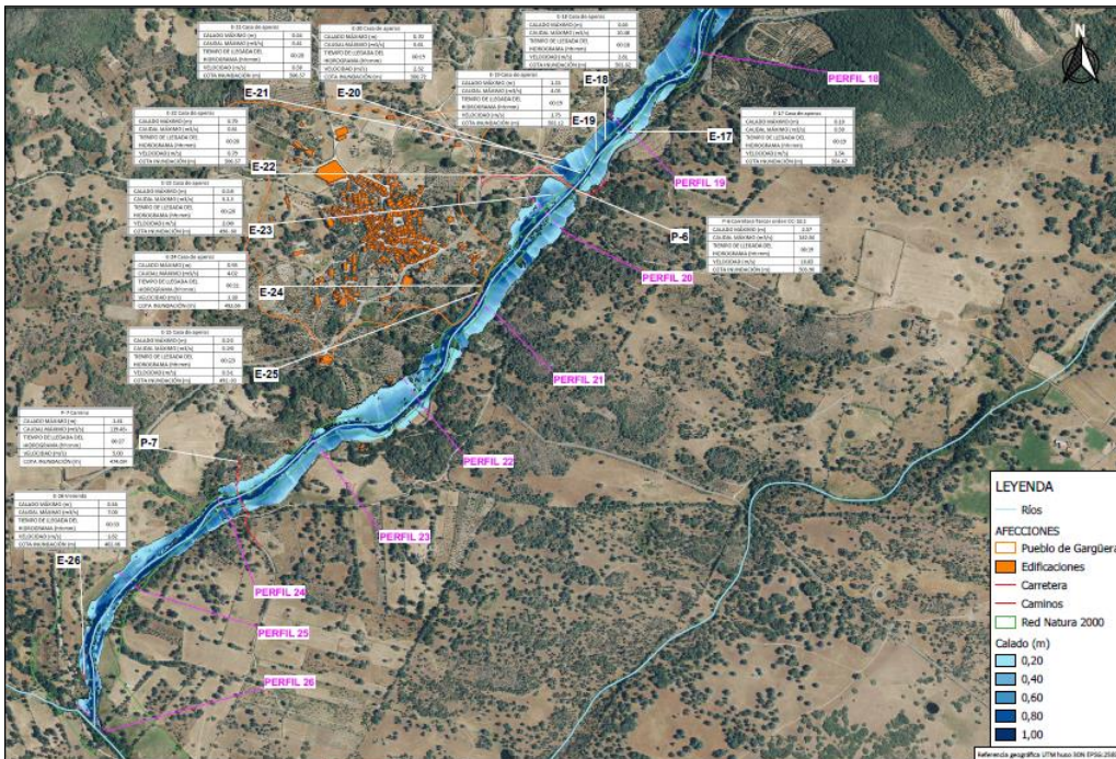
Ilustración 66. Calados máximos Balsa 1
