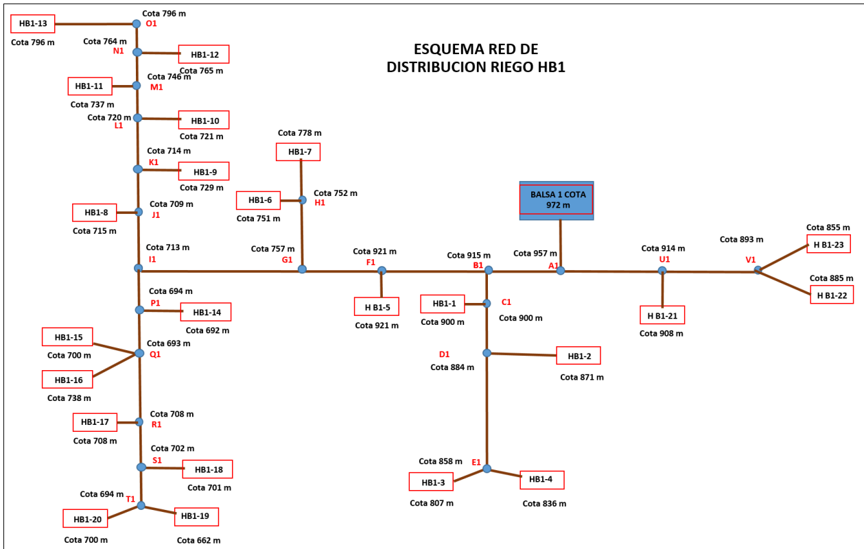
Esquema 7: Esquema Riego HB1
