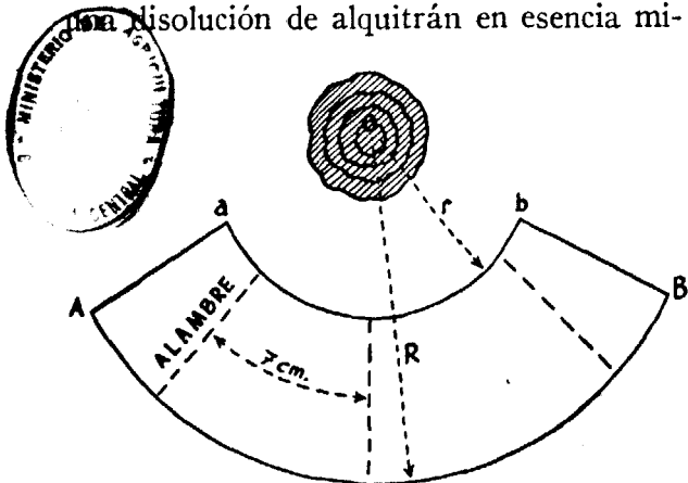
Fig. 17.—Detalle de la confección de una cubeta de tela (Servicio de Defensa de las Plantas, Rabat).
