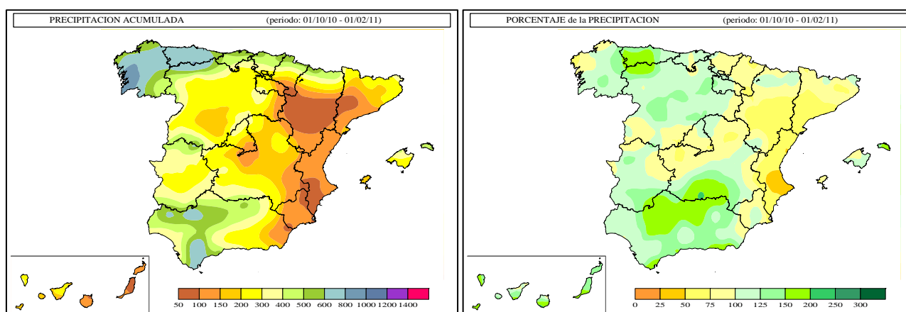
Figura 1. Precipitación acumulada y porcentaje de precipitación al 1 de febrero de 2011 (Fuente: AEMET)
