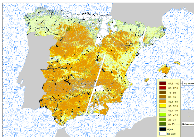
Figura 8. Índice normalizado de sequía en superficie (NSDI). Agosto 2010 (Fuente: MARM)
