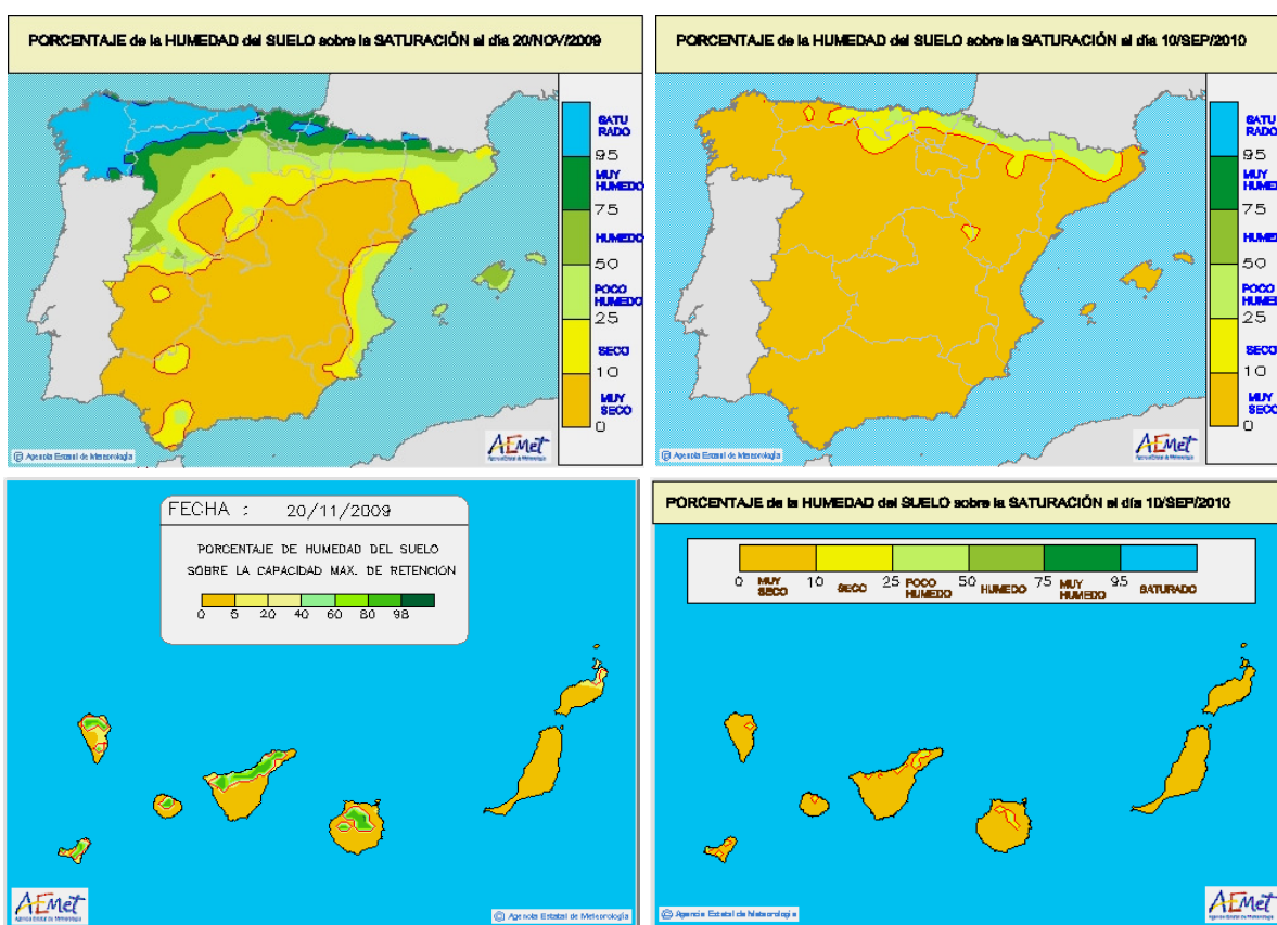
Figura 6. Porcentaje de la humedad del suelo sobre la saturación (Comparativa de la evolución entre el 20 de noviembre de 2009 y el 10 de septiembre de 2010) (Fuente: AEMET)
