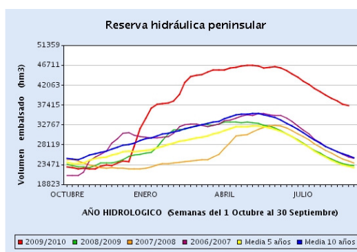
Figura 2. Reserva hidráulica total – semana del 14 al 21 de septiembre de 2010 (Fuente: Boletín Hidrológico)
