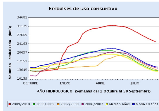
Figura 4. Reserva hidráulica Usos Consuntivos – semana del 14 al 21 de septiembre de 2010 (Fuente: Boletín Hidrológico)
