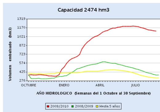
Figura 10. Volumen embalsado en la cabecera del Tajo a 21 de septiembre de 2010 (Fuente: Boletín Hidrológico)
