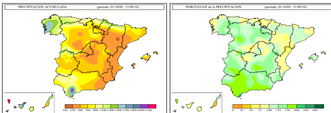
Figura 1. Precipitación acumulada y porcentaje de precipitación al 21 de septiembre de 2010 (Fuente: AEMET)
