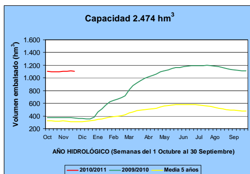
Figura 7. Volumen embalsado en la cabecera del Tajo a 23 de noviembre de 2010 (Fuente: Boletín Hidrológico)
