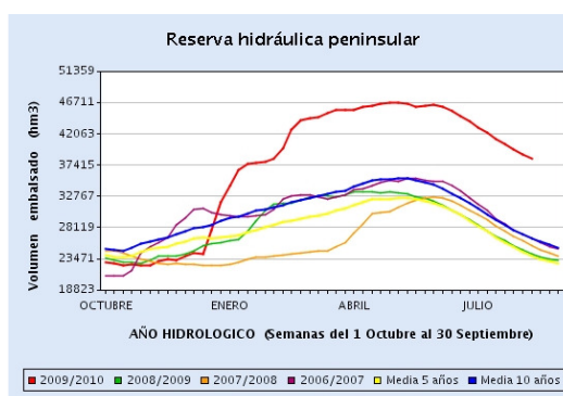
Figura 2. Reserva hidráulica total – semana del 7 al 14 de septiembre de 2010 (Fuente: Boletín Hidrológico)
