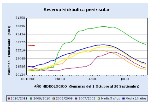
Figura 2. Reserva hidráulica total – semana del 19 al 26 de octubre de 2010 (Fuente: Boletín Hidrológico)
