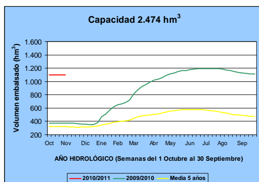
Figura 10. Volumen embalsado en la cabecera del Tajo a 2 de noviembre de 2010 (Fuente: Boletín Hidrológico)
