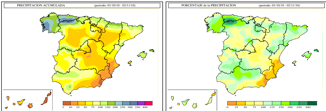
Figura 1. Precipitación acumulada y porcentaje de precipitación al 2 de noviembre de 2010 (Fuente: AEMET)
