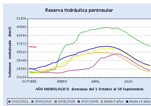
Figura 2. Reserva hidráulica total – semana del 26 de octubre al 2 de noviembre de 2010 (Fuente: Boletín Hidrológico)
