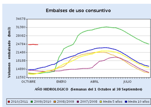
Figura 4. Reserva hidráulica Usos Consuntivos – semana del 26 de octubre al 2 de noviembre de 2010 (Fuente: Boletín Hidrológico)
