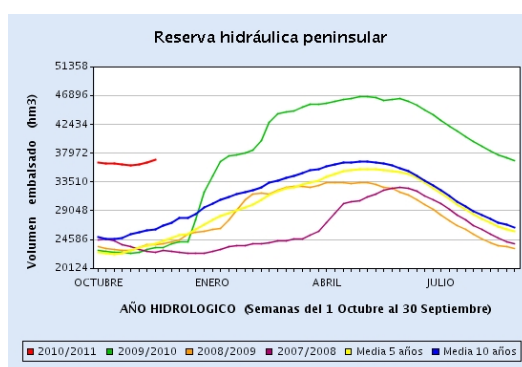
Figura 2. Reserva hidráulica total – semana del 23 al 30 de noviembre de 2010 (Fuente: Boletín Hidrológico)
