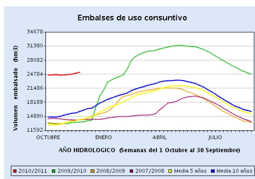
Figura 4. Reserva hidráulica Usos Consuntivos – semana del 23 al 30 de noviembre de 2010 (Fuente: Boletín Hidrológico)
