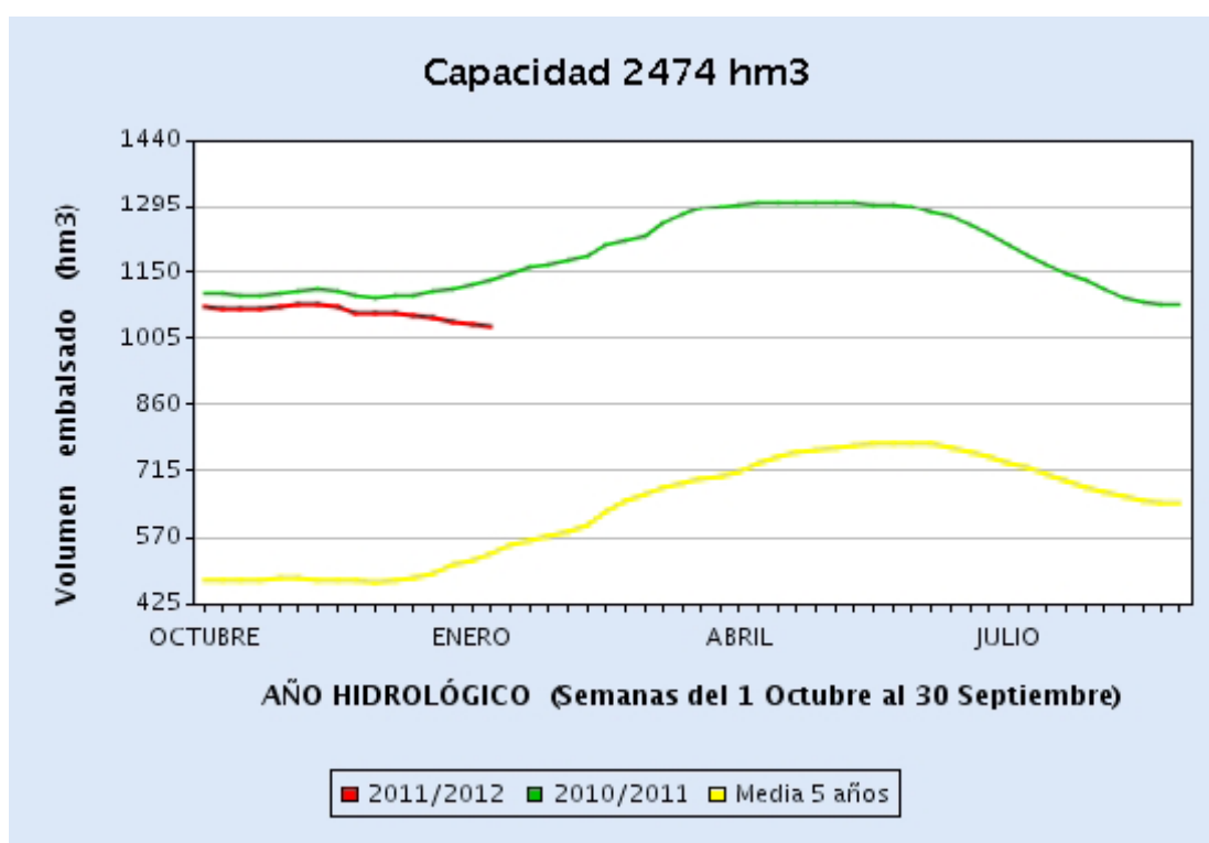
Figura 7. Volumen embalsado en la cabecera del Tajo a 17 de enero de 2012 (Fuente: Boletín Hidrológico)
