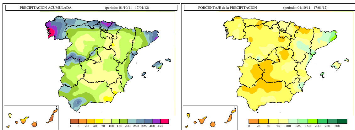
Figura 1. Precipitación acumulada en mm y porcentaje de precipitación (media 1970/2000) a 17 de enero de 2012 (Fuente: AEMET)
