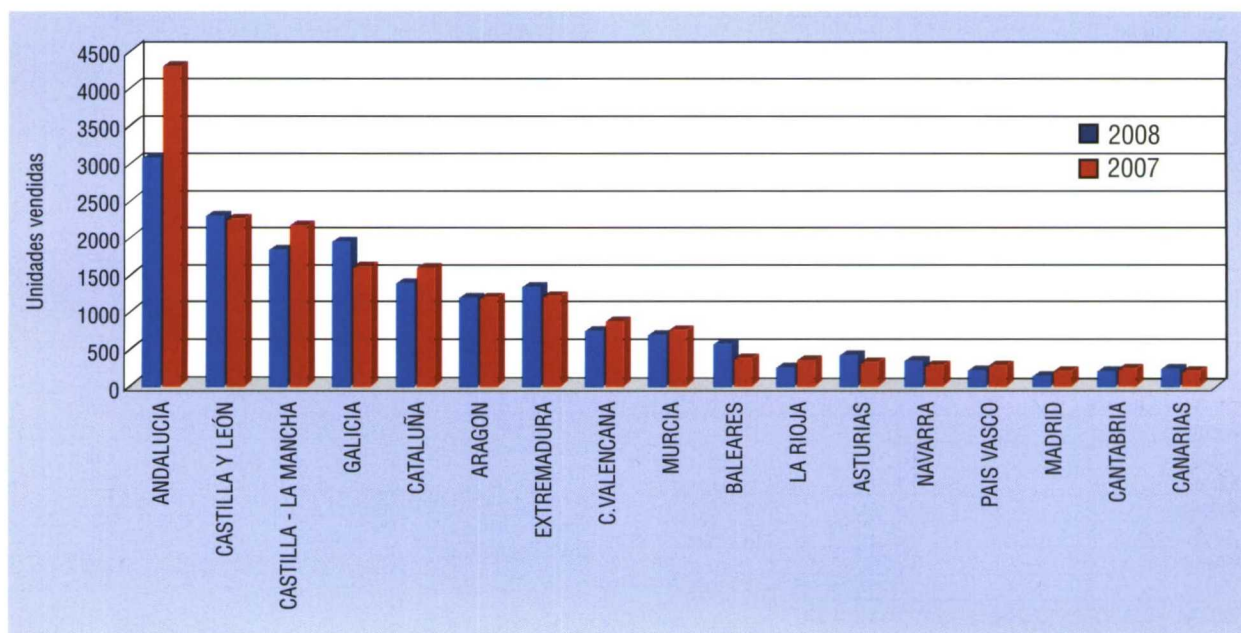
COMPARATIVA DE VENTAS DE TRACTORES, POR CCAA, DURANTE EL BIENIO 2007-2008
