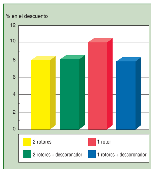
GRÁFICO 1. RESIDUO EN EL DESCUENTO EN FUNCIÓN DEL DESCORONADO
