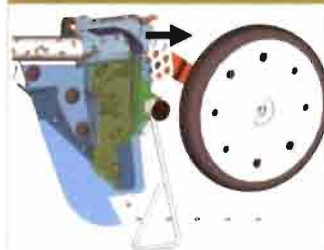
KUHN: Elemento sembrador en cascada ACCURA
