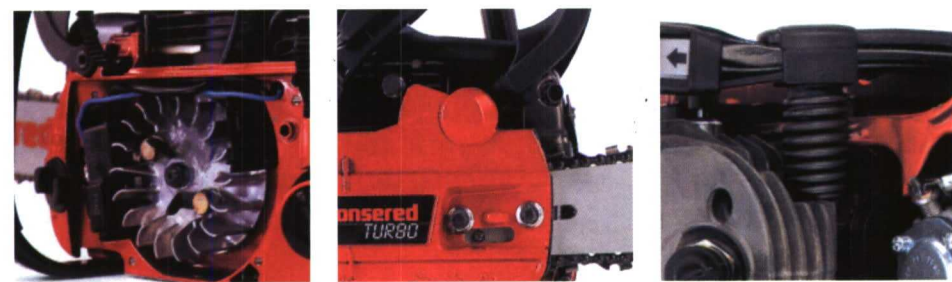
Una mejor purificación del aire, un nuevo tensor de cadena, de montaje lateral, y muelles de acero para amortiguar vibraciones, son algunas de las características básicas de este modelo.
