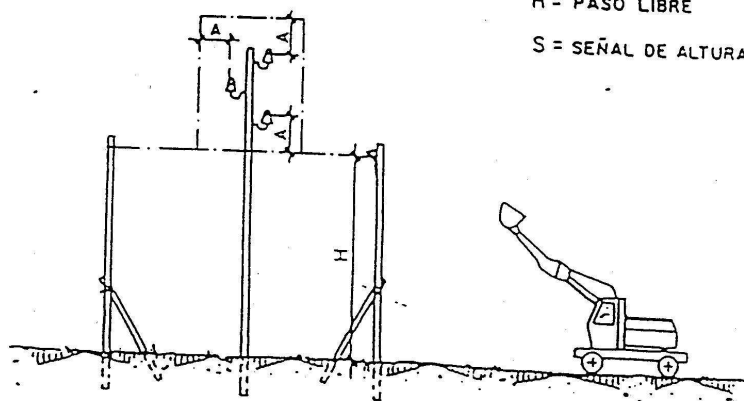
DETALLE - 2
