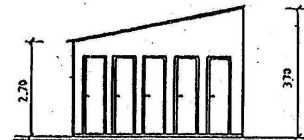
SECCION A-A'
