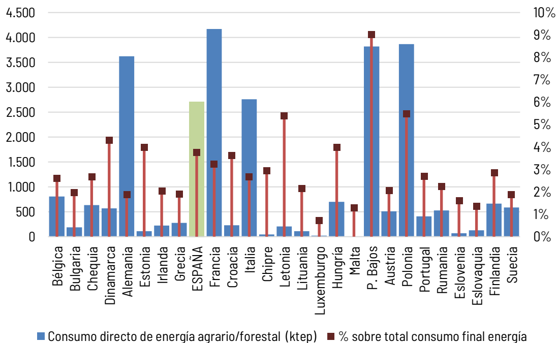
Gráfico 1.3.1. Uso directo de energía en el sector agrario/forestal (ktep) y su cuota (%) de participación en el consumo final, en la UE27 2020.
