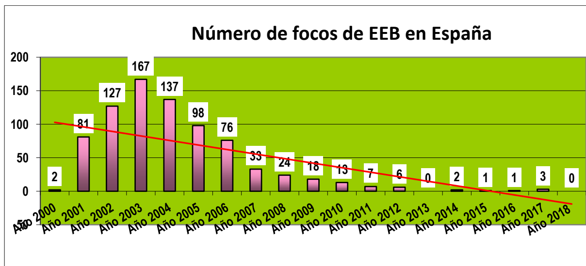
Gráfica B2: Evolución de los focos de EEB detectados en España. Periodo 2000- 31 diciembre 2018
