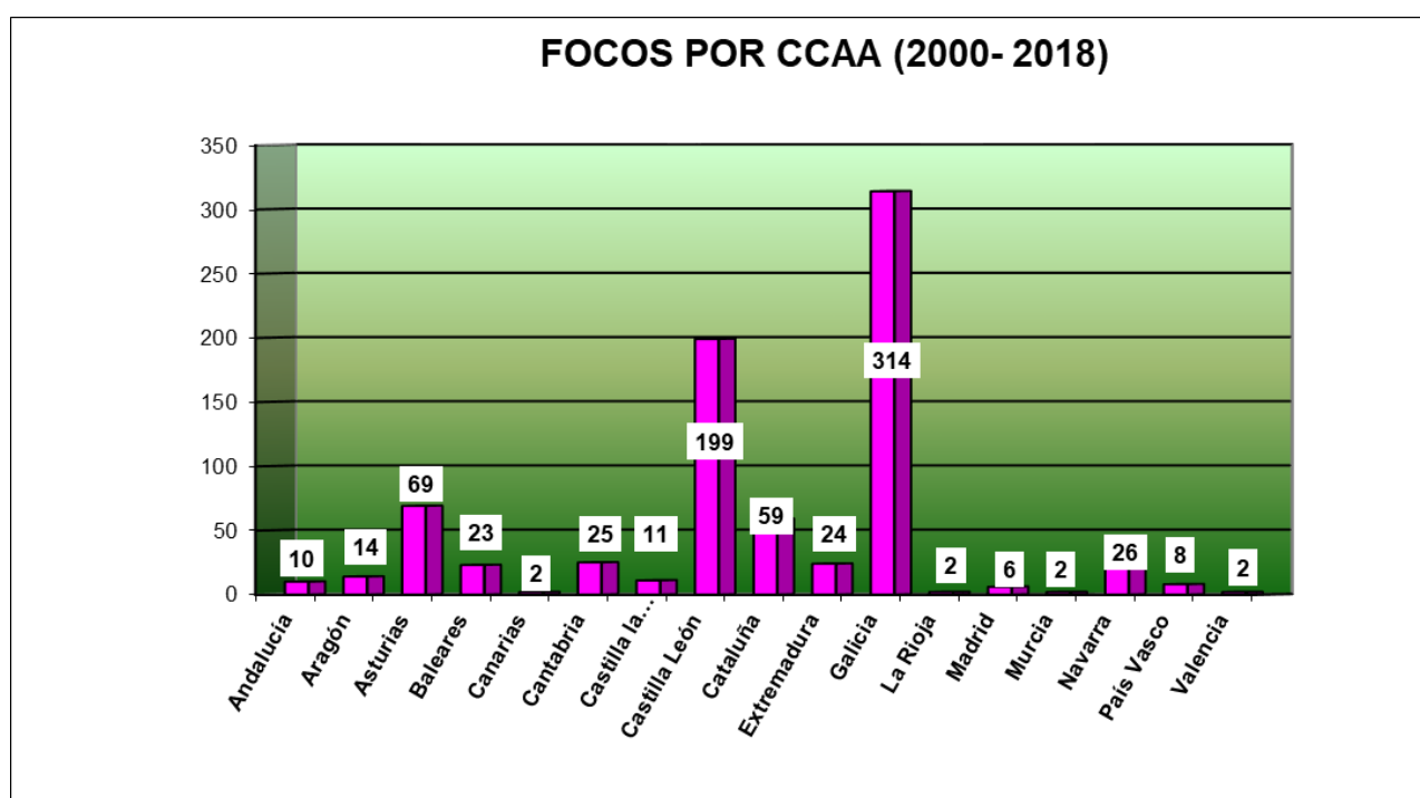
Gráfica B3: Distribución de focos por CCAA. Periodo 2000- 31 diciembre 2018
