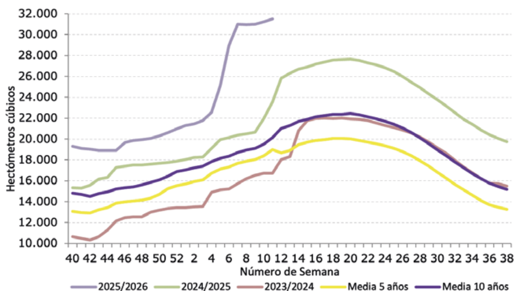
Gráfico 1.3.1. Evolución de la reserva de los embalses de uso consuntivo. Miles de hm 3 . Año hidrológico de 1 de octubre a 30 de septiembre.
