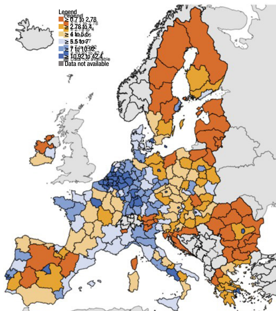
Mapa 1.2.2. Porcentaje de suelo ocupado por áreas artificiales. Porcentaje sobre el total del suelo. 2022.
