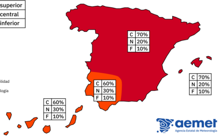
PROBABILIDAD DE LA CATEGORÍA MÁS PROBABLE DE TEMPERATURA JULIO - AGOSTO - SEPTIEMBRE 2026
